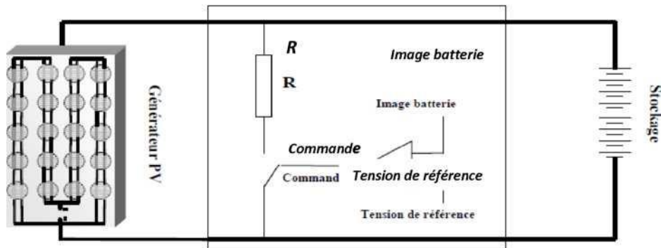
Figure I.8 : Régulateur parallèle
