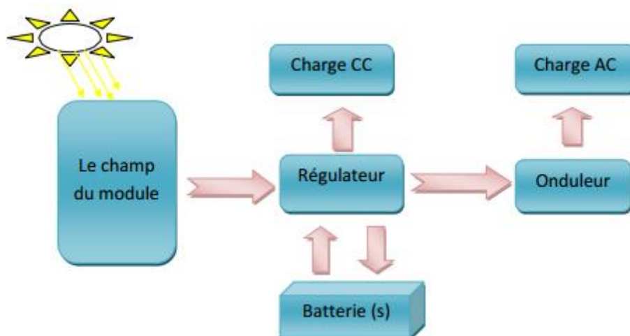
Figure I.1: Schéma synoptique d'un système photovoltaïque autonome.
