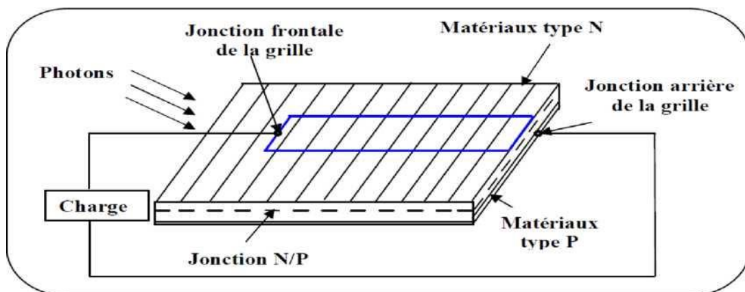
Figure I.3 : principe de conversion de l'énergie solaire en énergie électrique par cellule
