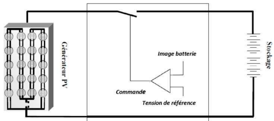
Figure I.9 : Régulateur série
