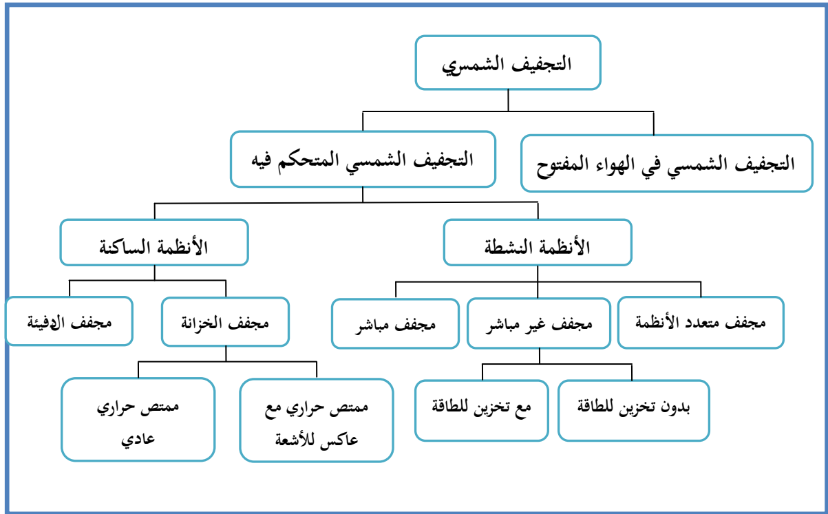
شكل رقم (1): أنظمة التجفيف بالطاقة الشمسية.
