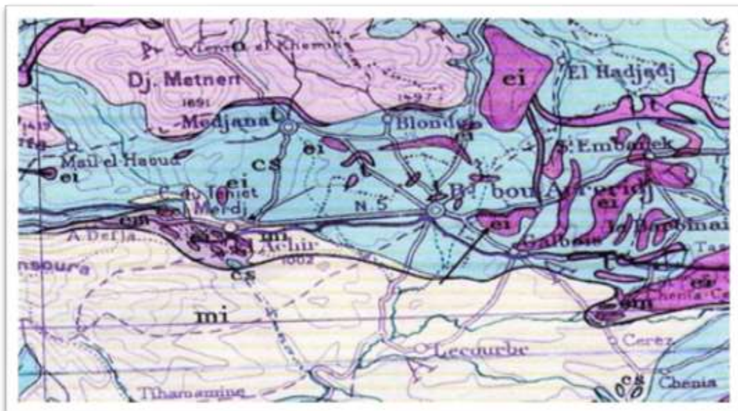
الشكل (9): جيولوجية شمال الجزائر
