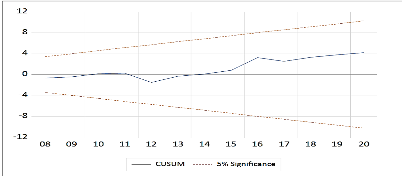
الشكل رقم(16): إختبار المجموع التراكمي للبواقي المعاودة (CUSUM)
