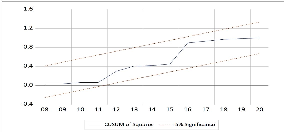
الشكل رقم(17): إختبار المجموع التراكمي لمربعات البواقي المعاودة (CUSUM Of Squares)
