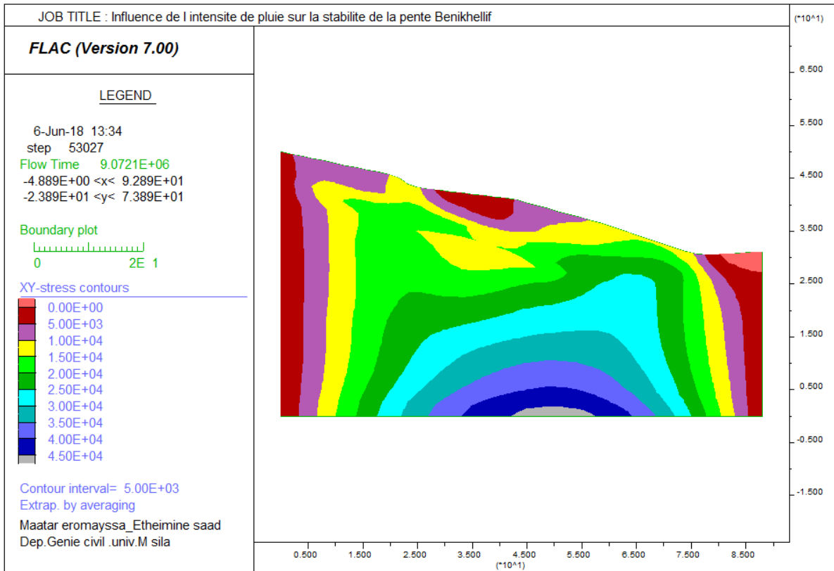
Figure IV.10 : Distributions des contraintes tangentielles (conditions initiales)
