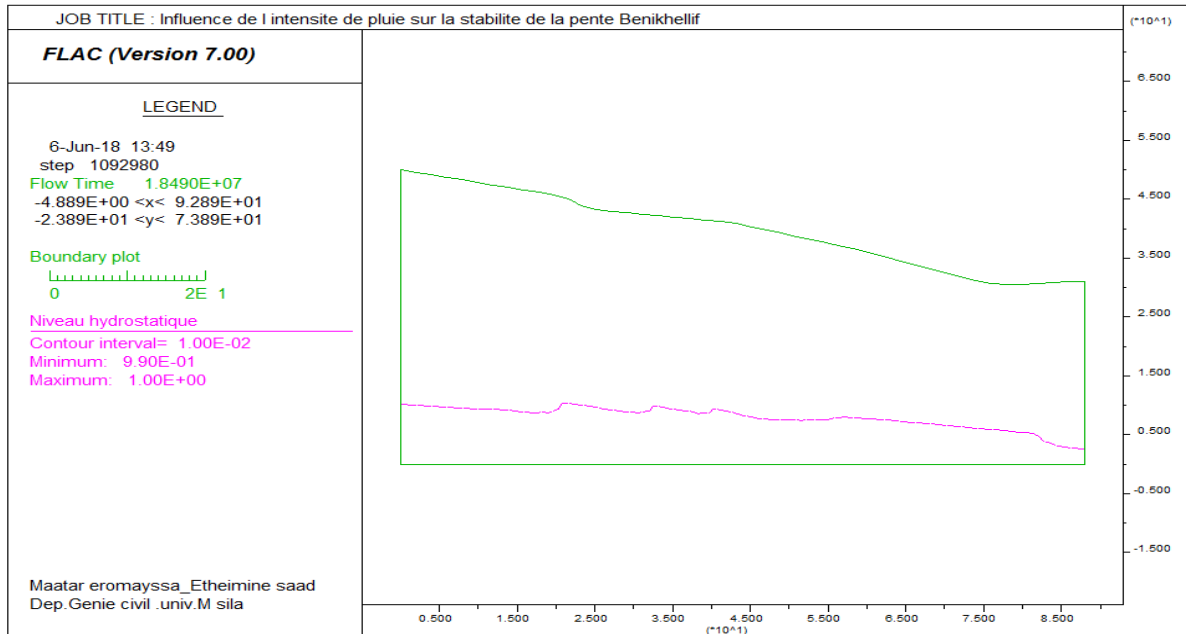
Figure IV.18 : Niveau hydrostatique (Deuxième évènement de Pluie)
