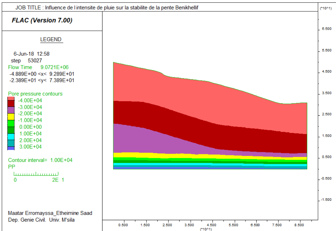
Figure IV.4 : Distribution de la pression interstitielle (conditions initiales)
