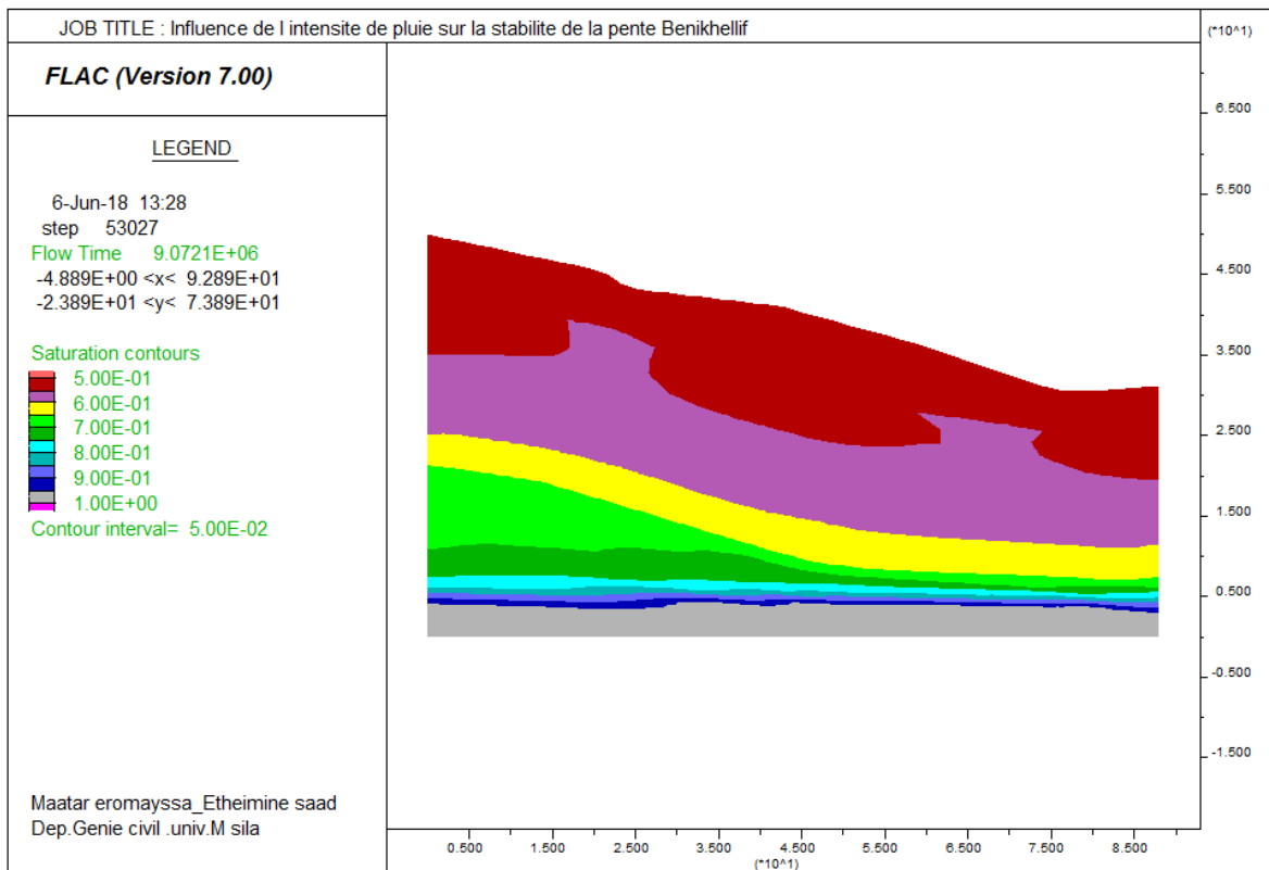
Figure IV.5 Distribution de la saturation résultante (conditions initiales)
