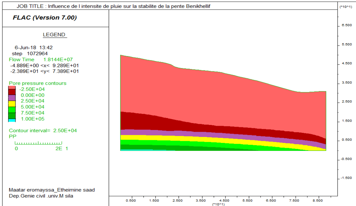
Figure IV.12: Pression interstitielle (Premier évènement de Pluie)
