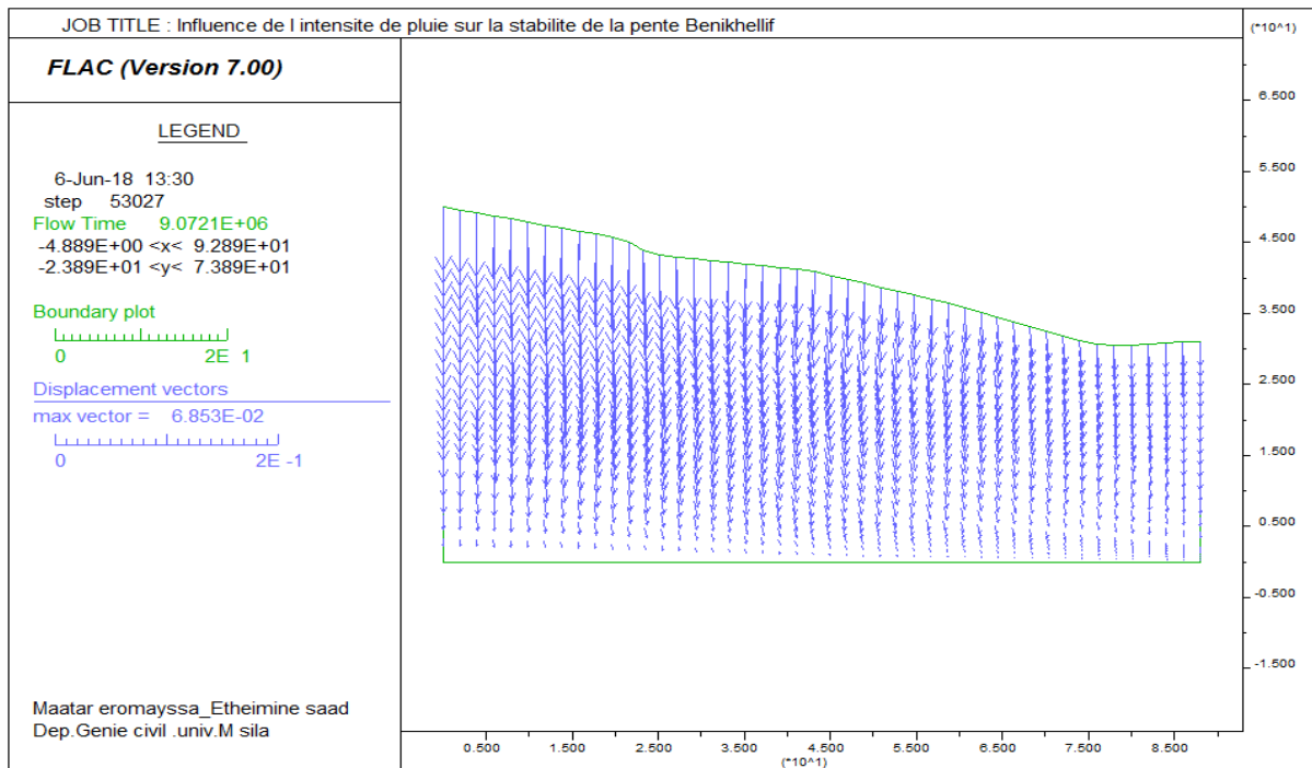
Figure IV.7 : Déplacements totaux (conditions initiales)
