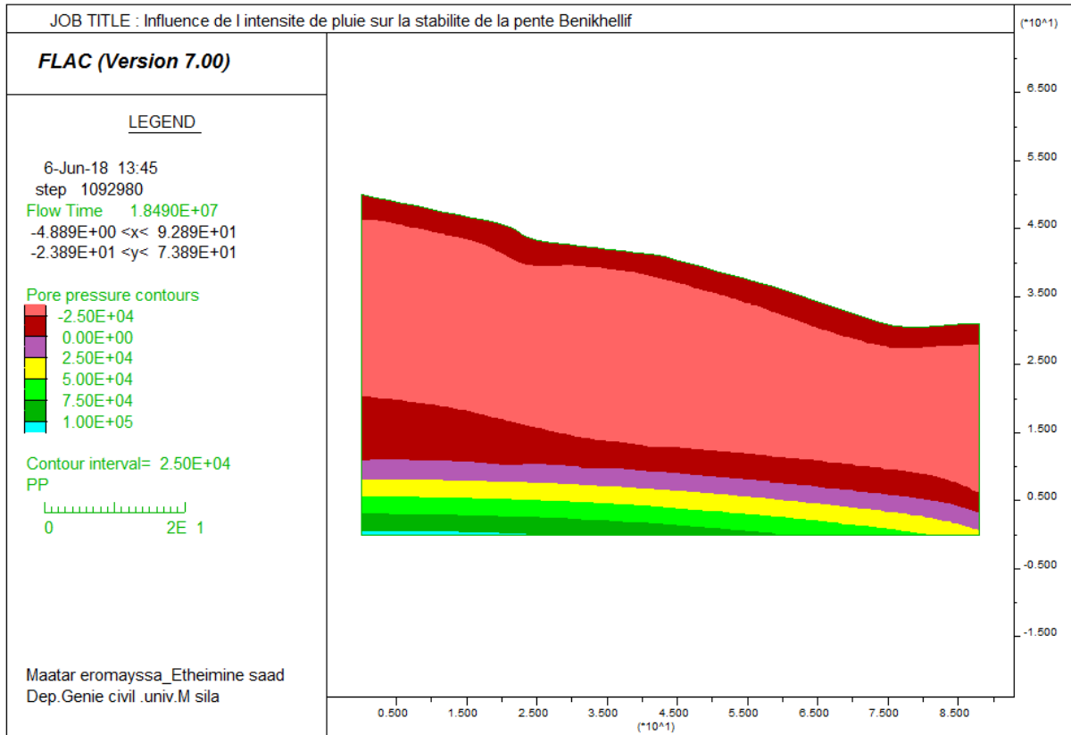
Figure IV.16 : Pressions interstitielles (Deuxième évènement de Pluie)
