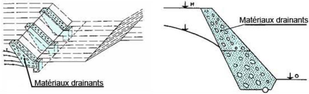
Figure 1.4 : éperon drainant et masque drainant
