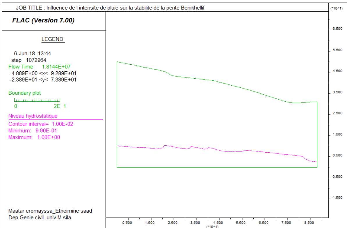
Figure IV.14: Niveau hydrostatique (Premier événement de pluie)
