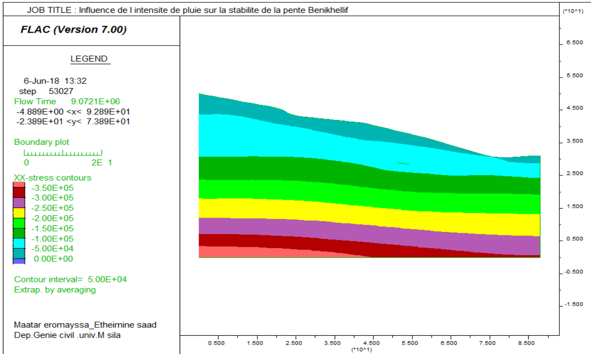
Figure IV.8 Distributions des contraintes horizontales (conditions initiales)
