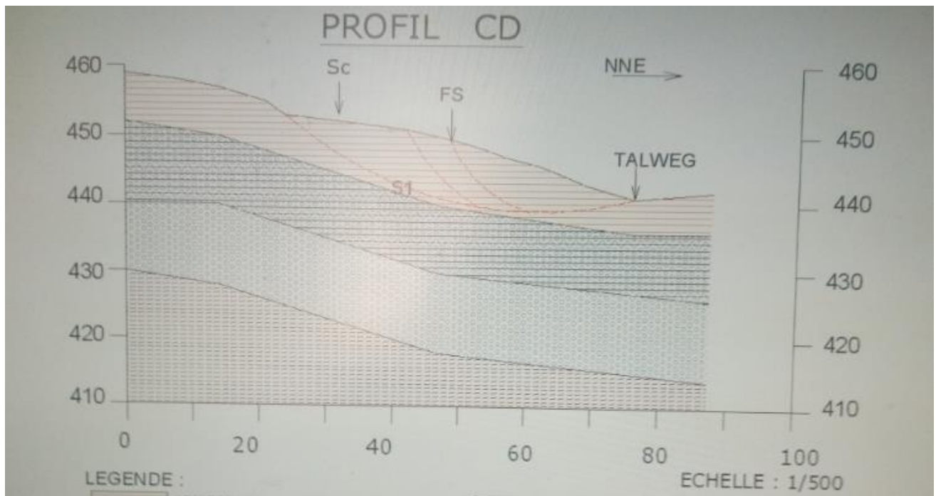
Figure III.2 : le profil CD étudié
