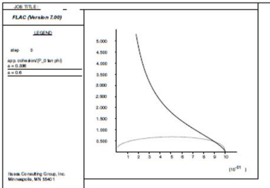
Figure IV.2 : courbe de cohésion C_c / (P_0 \tan \phi) en fonction de saturation effective S_e pour a=0.336 et a=0.6
