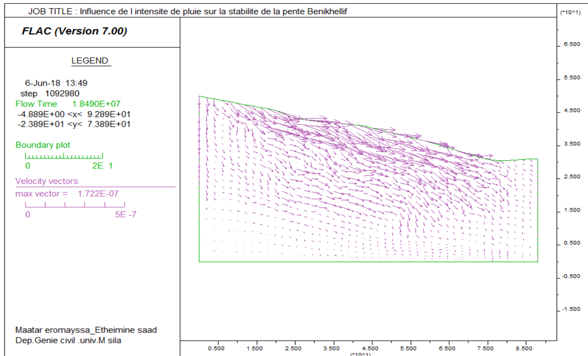
Figure IV.19 : Vitesses de déplacements (Deuxième évènement de Pluie)
