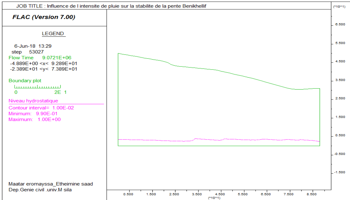
Figure IV.6 : Niveau hydrostatique (niveau de saturation totale) (conditions initiales)
