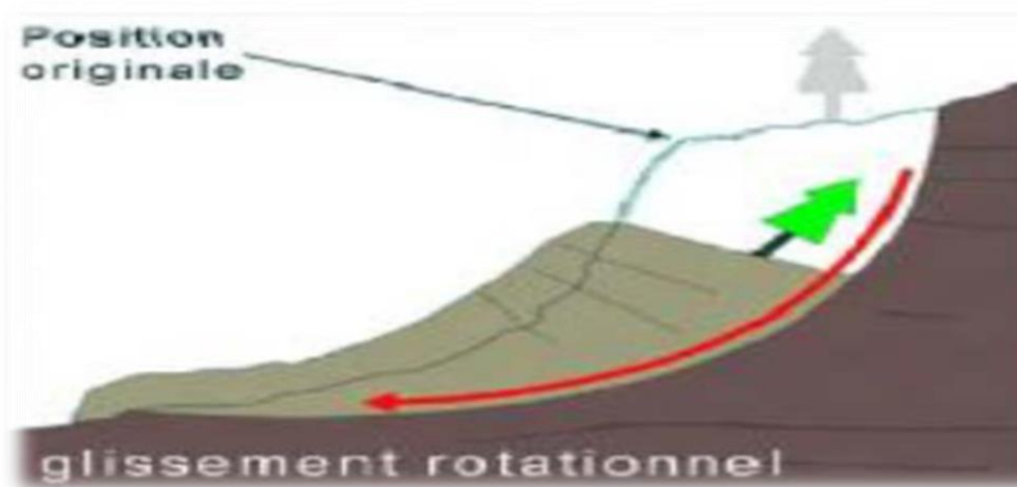
Figure I.2 : glissement rotationnel simple
