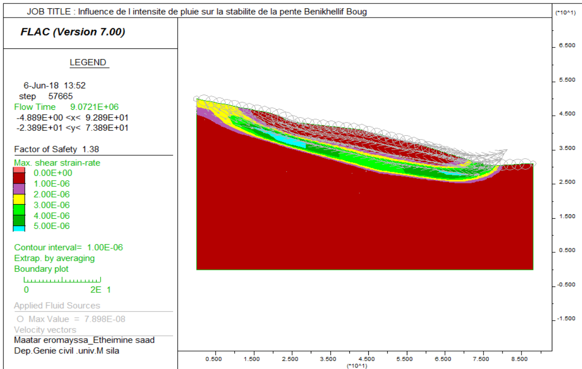
Figure IV.11 : Facteur de sécurité (conditions initiales)
