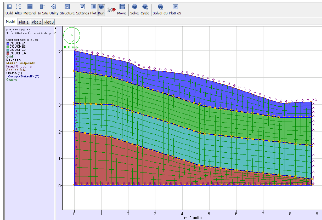
Figure IV.3 : La géométrie de la pente et la grille FLAC pour les simulations
