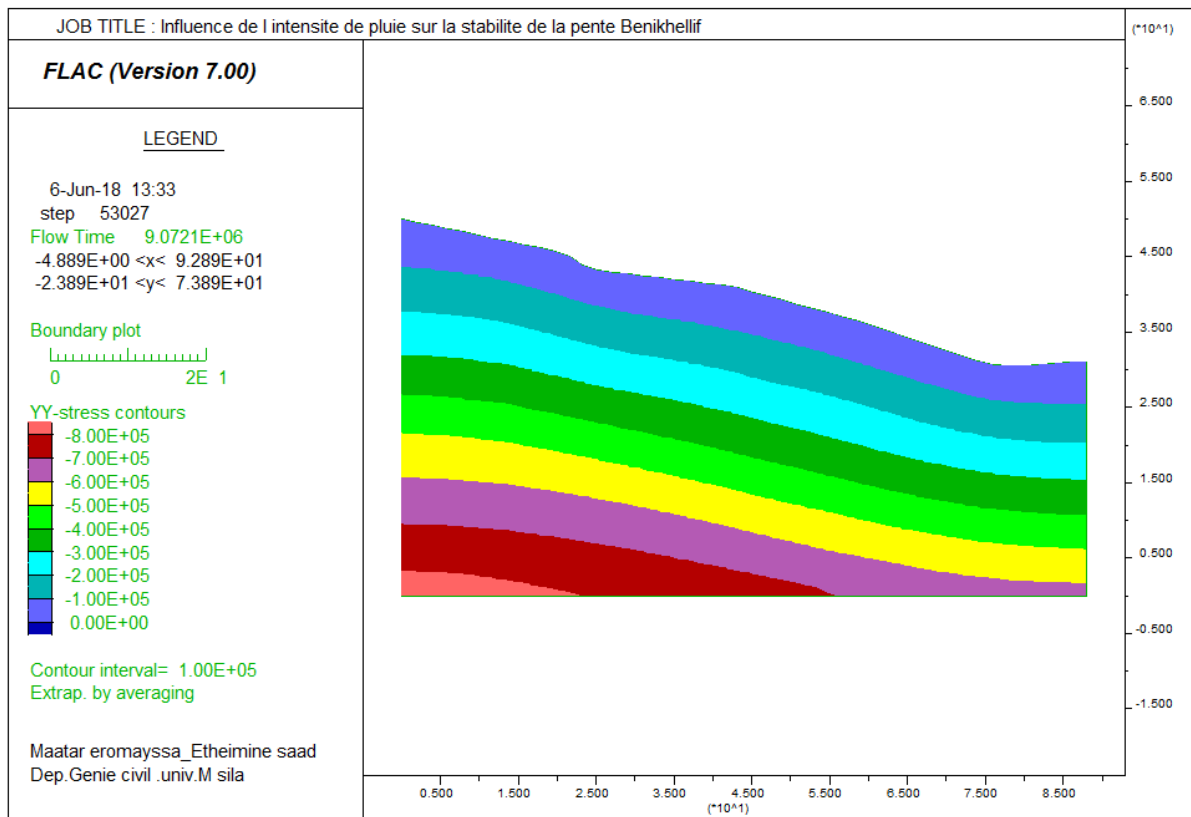
Figure IV.9 : Distributions des contraintes verticales (conditions initiales)
