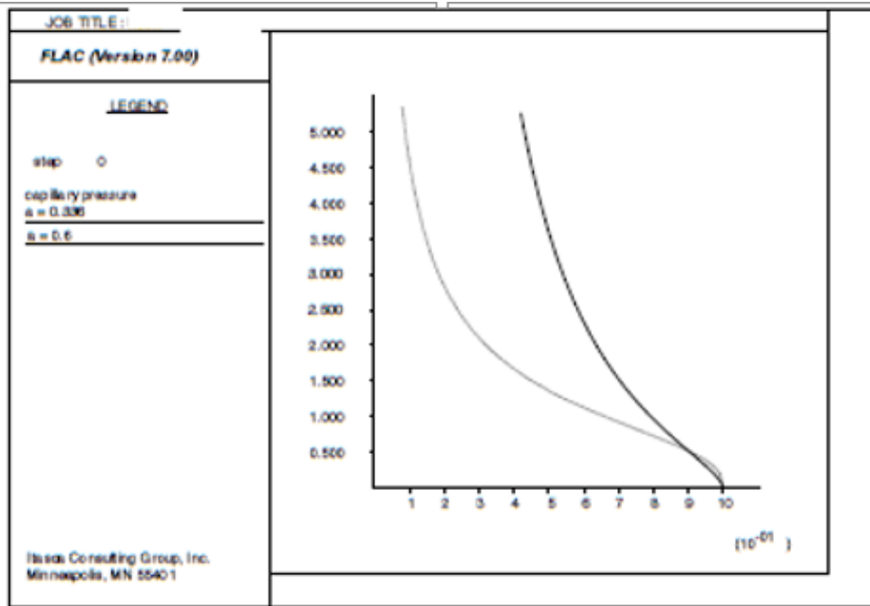
Figure IV.1 : courbe capillaire P_C / P_0 en fonction de la saturation effective S_e pour a=0.336 et a=0.6
