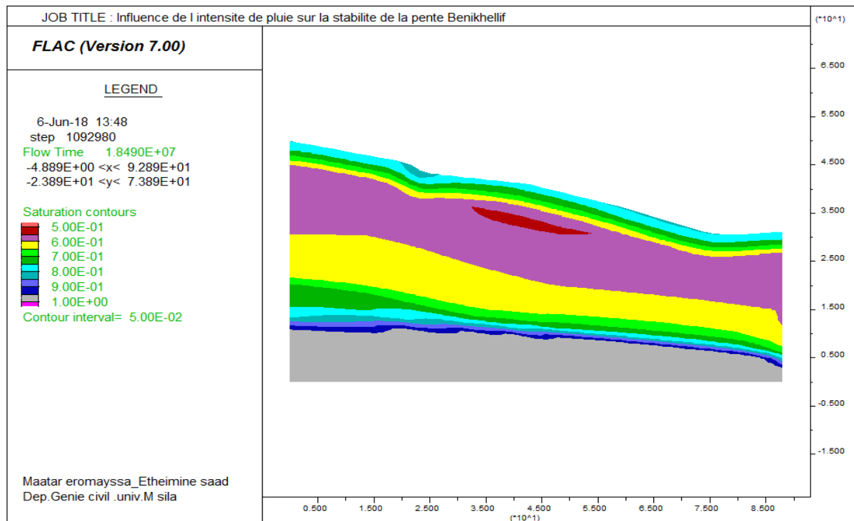
Figure IV.17 : Distribution de la saturation (Deuxième évènement de Pluie)
