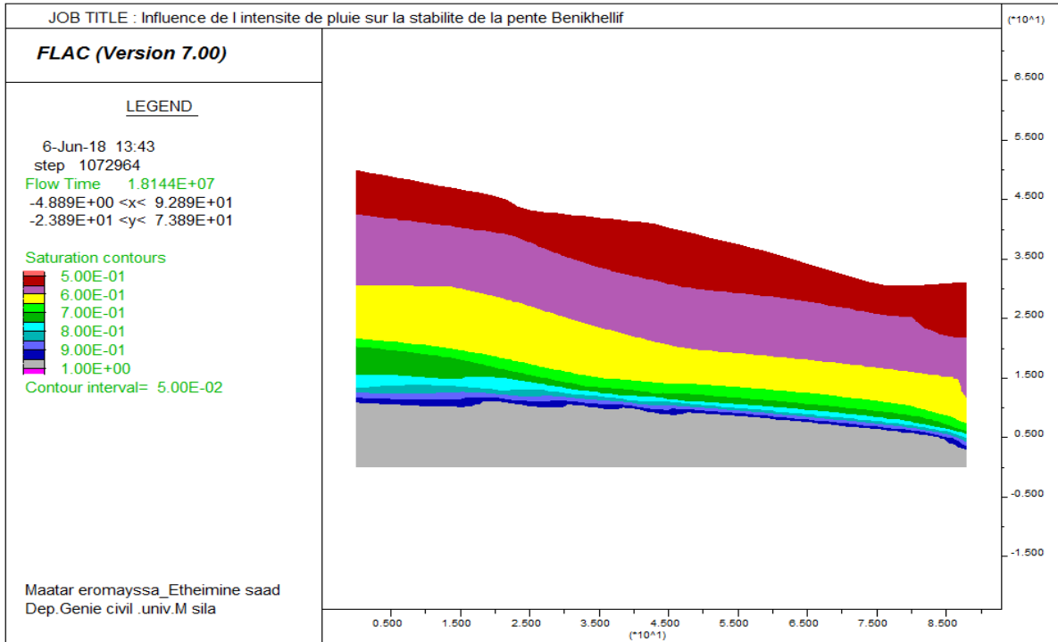
Figure IV.13: Distribution de la saturation (Premier événement de Pluie)
