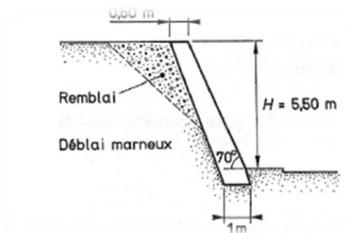
Figure1.14 : mur en Texsol
