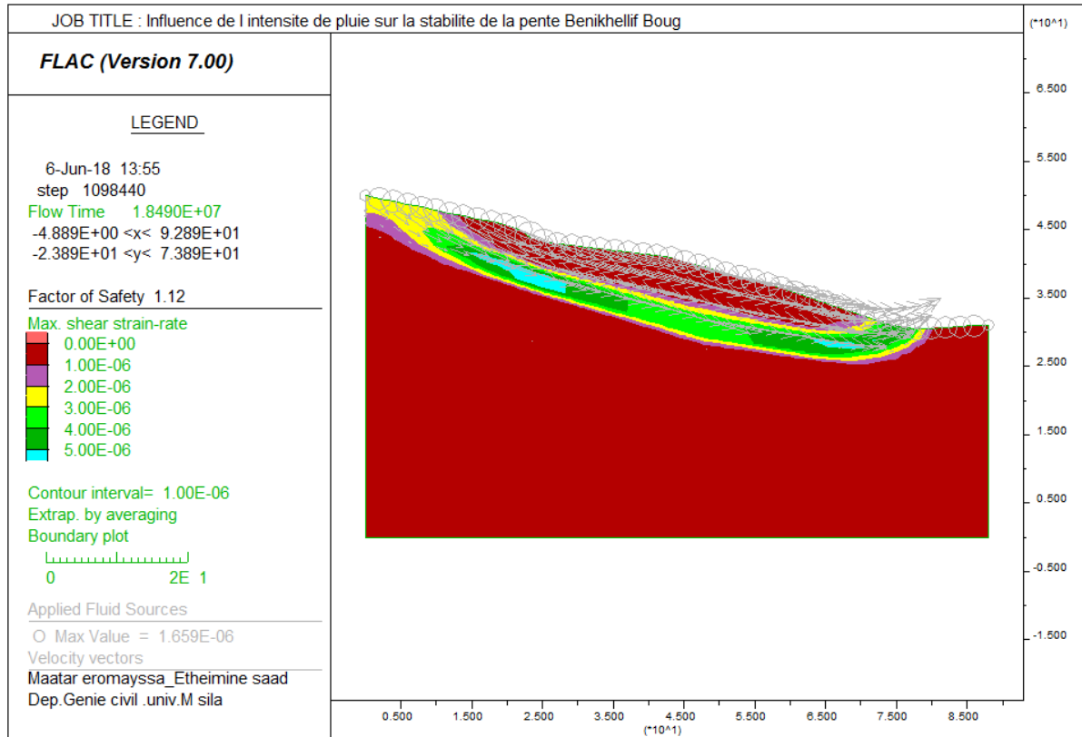
Figure IV.20 Facteur de sécurité (Deuxième évènement de Pluie)
