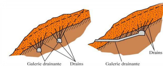
Figure 1.7 : Galerie drainante
