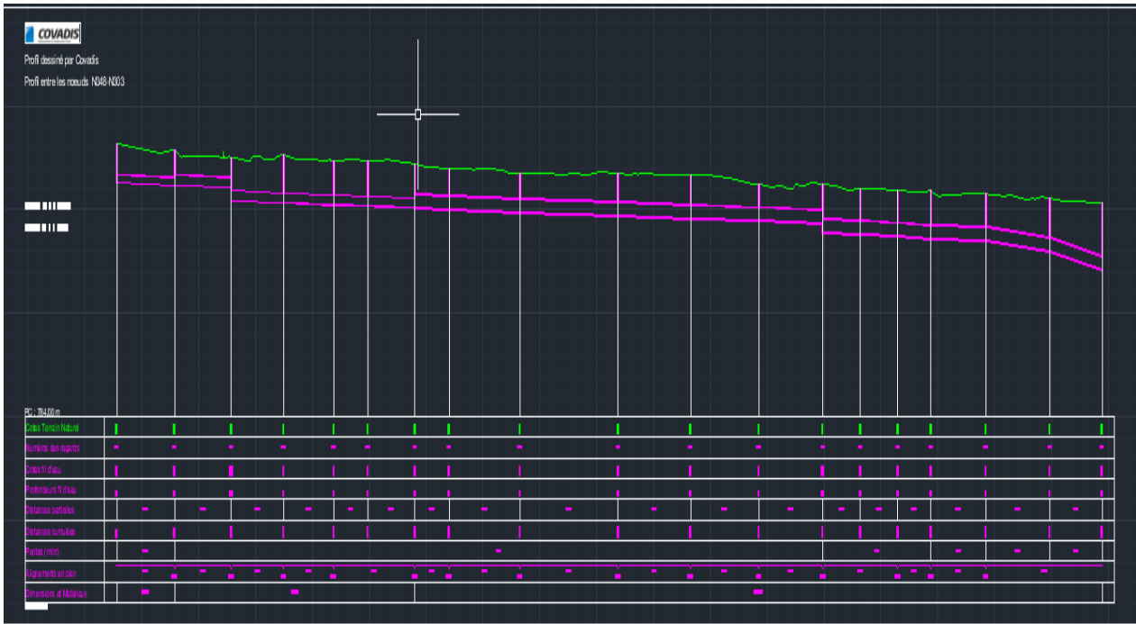
Figure01 : Profil en long entre les nœuds N348-N303
