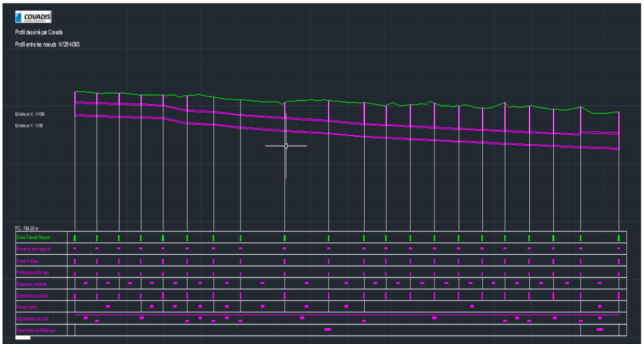
Figure02 : Profil en long entre les nœuds N126-N303
