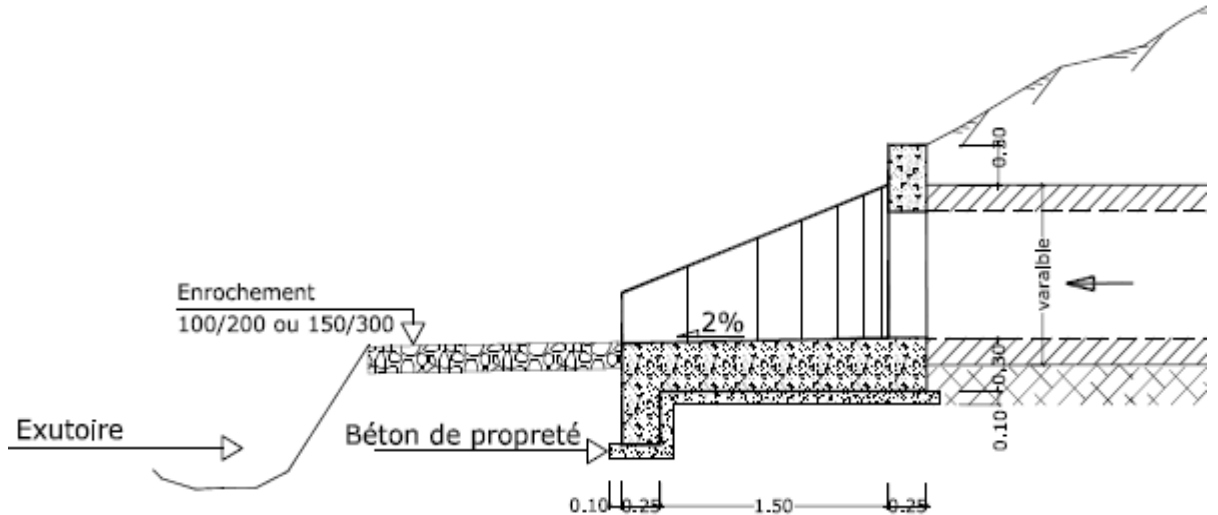
Figure VI*8 : ouvrage de rejet vu de gauche.
