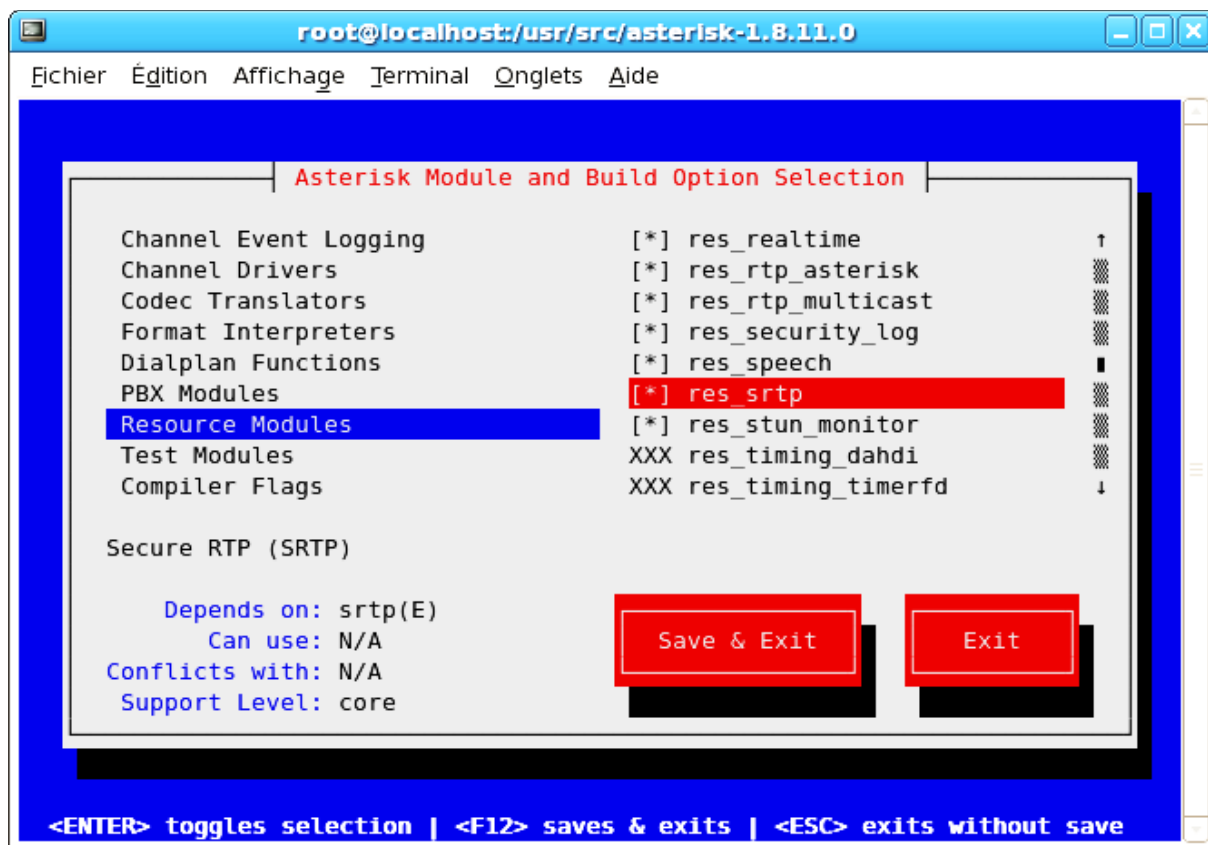
Figure 25 : Ajoute de SRTP sur Asterisk
