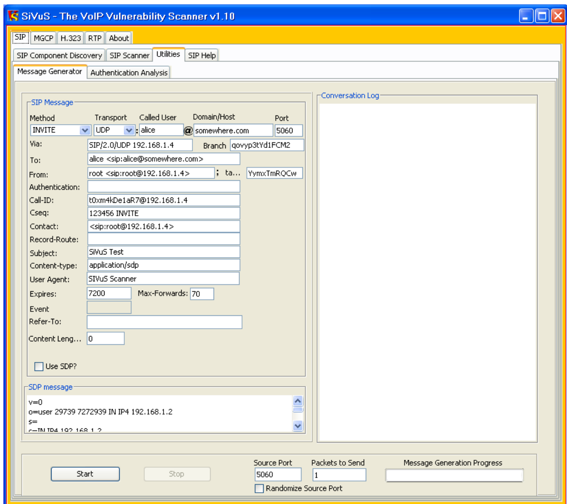
Figure 21 : SiVuS : fenêtre de génération de message
