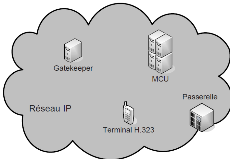
Figure 2 : Les composants de l'architecture H.323 [5]
