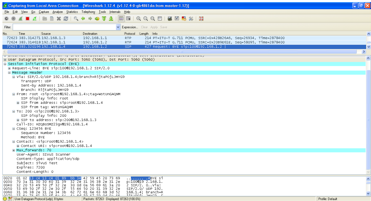
Figure 24 : Message envoyé par SiVus apparaît dans Wireshark
