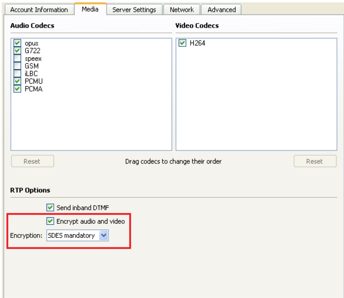
Figure 26 : Configuration de SRTP dans Blink
