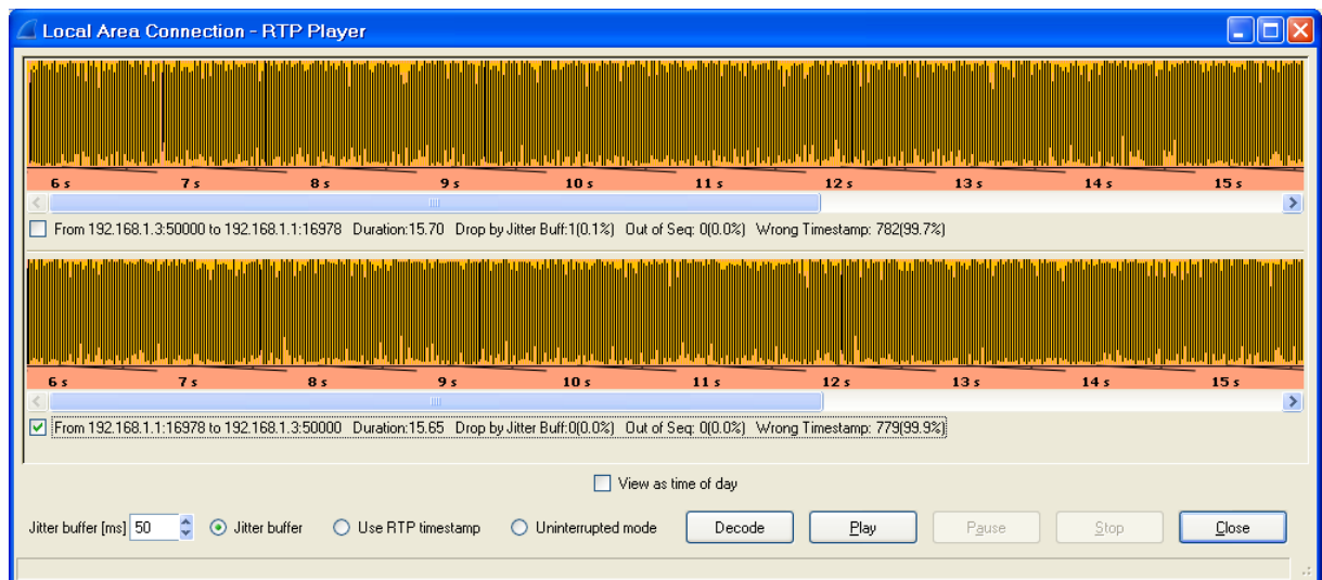
Figure 28 : Communication téléphonique par SRTP décodé
