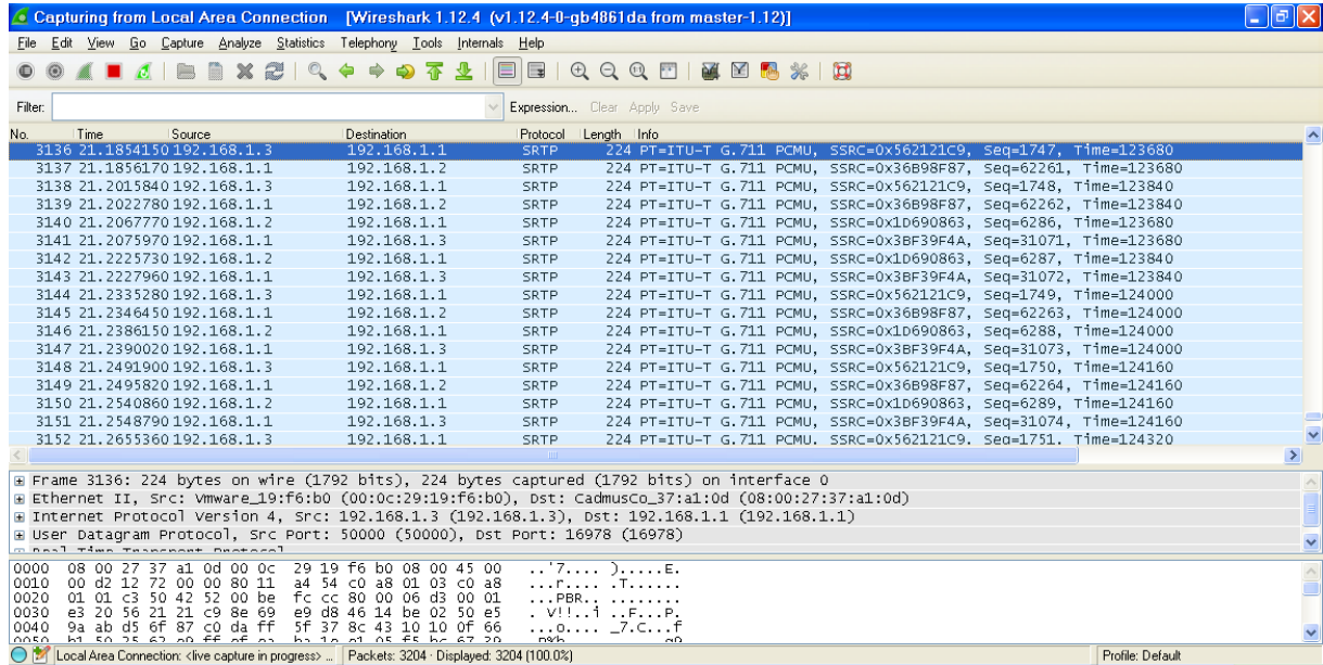
Figure 27 : Communication téléphonique à partir de SRTP
