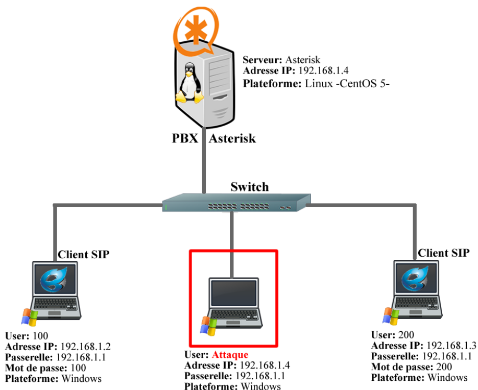
Figure 12 : Architecture du réseau VoIP à réaliser
