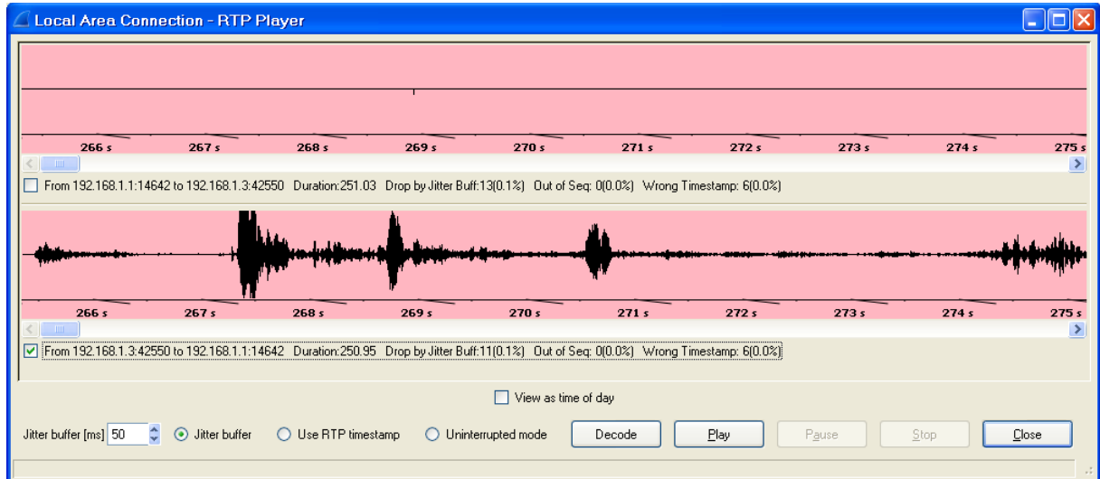
Figure 20 : Communication téléphonique décodé
