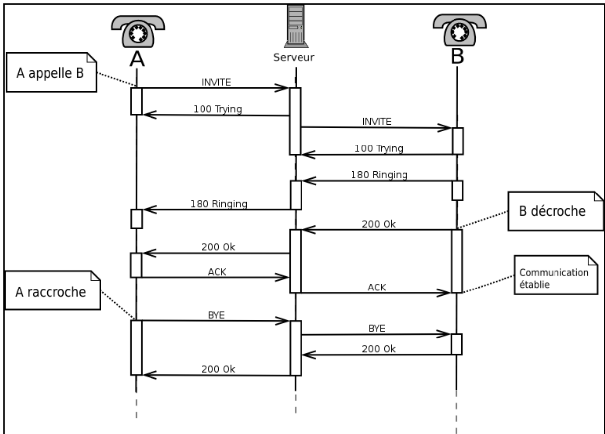
Figure 8 : Session SIP à travers un proxy [6]
