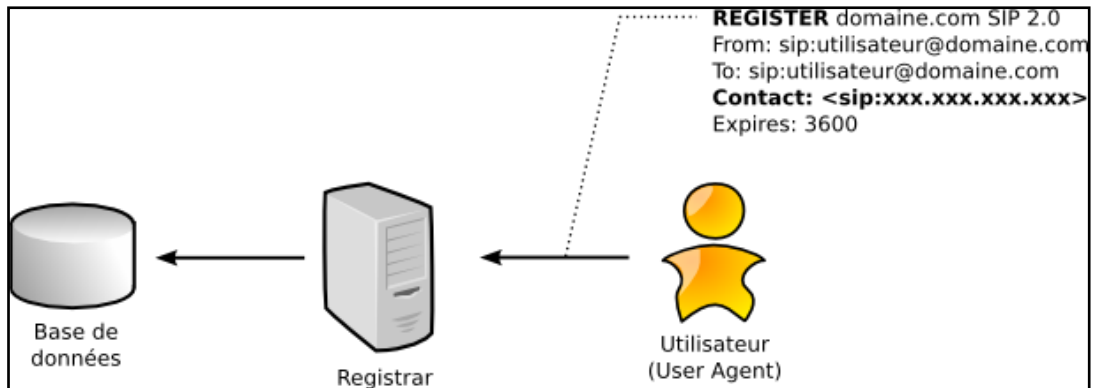
Figure 6 : Enregistrement d'un utilisateur [6]
