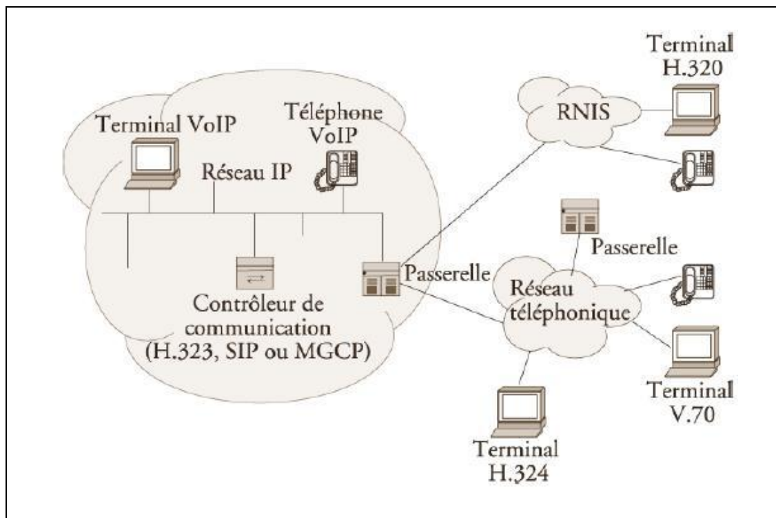
Figure 1 : Architecture générale de la voix sur IP [2]
