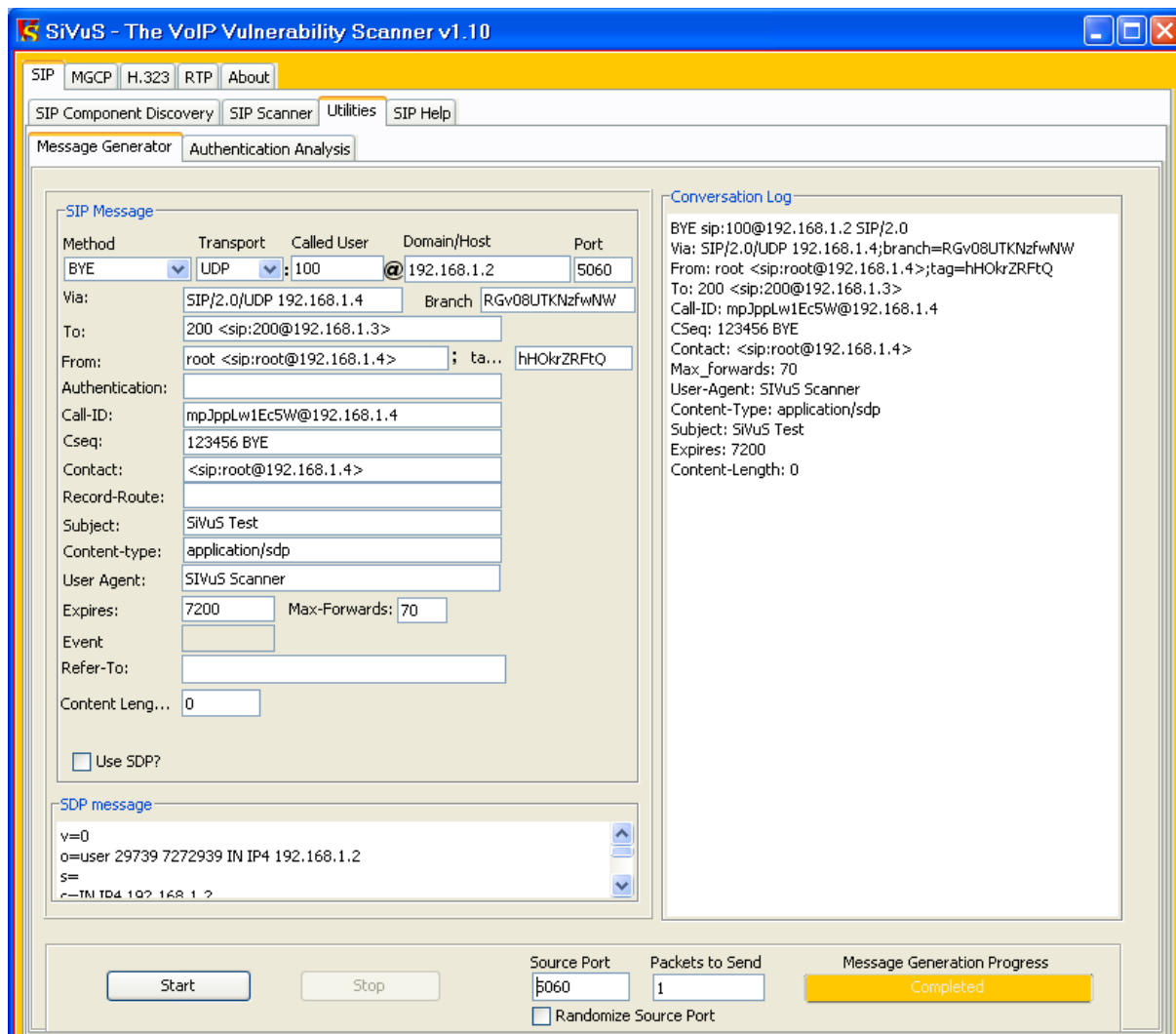
Figure 23 : Génération de message de type BYE
