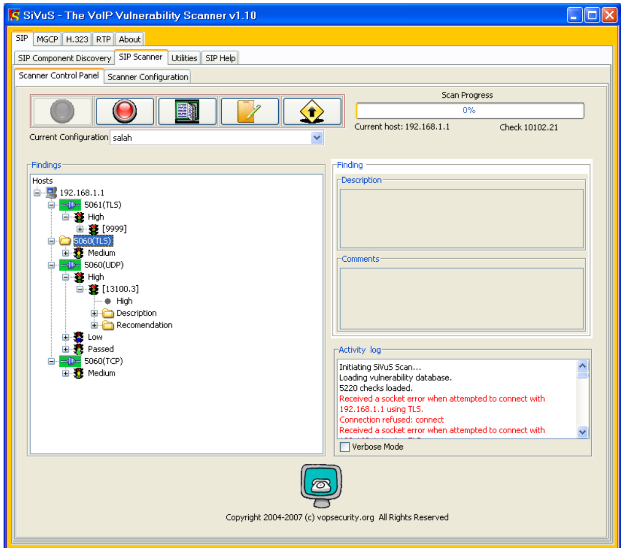
Figure 22 : Scanne de la machine 192.168.1.1
