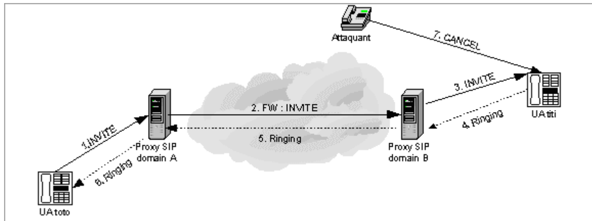
Figure 9 : Attaque DoS via une requête CANCEL [9]
