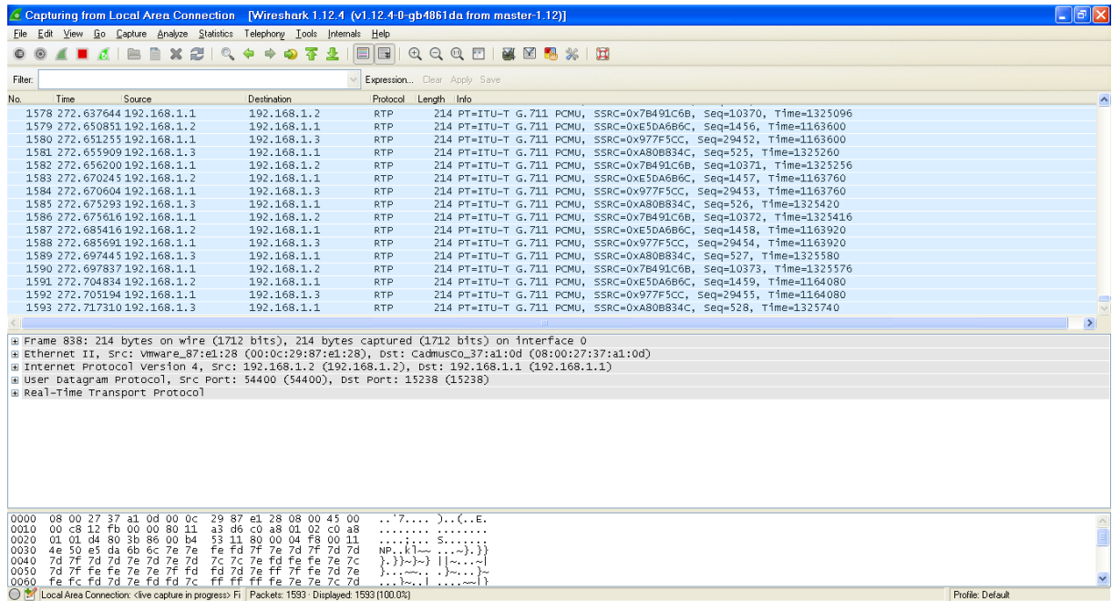
Figure 16 : Capture d'une communication téléphonique
