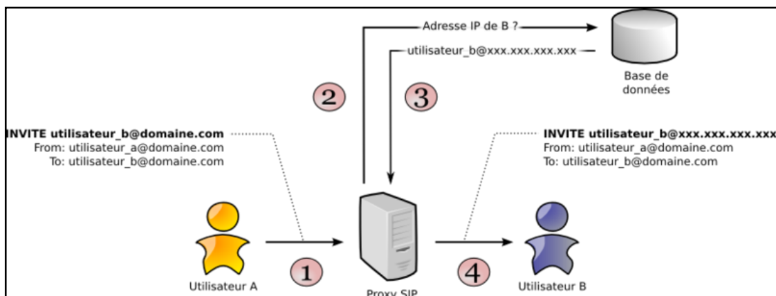
Figure 7 : Principe du protocole SIP [6]
