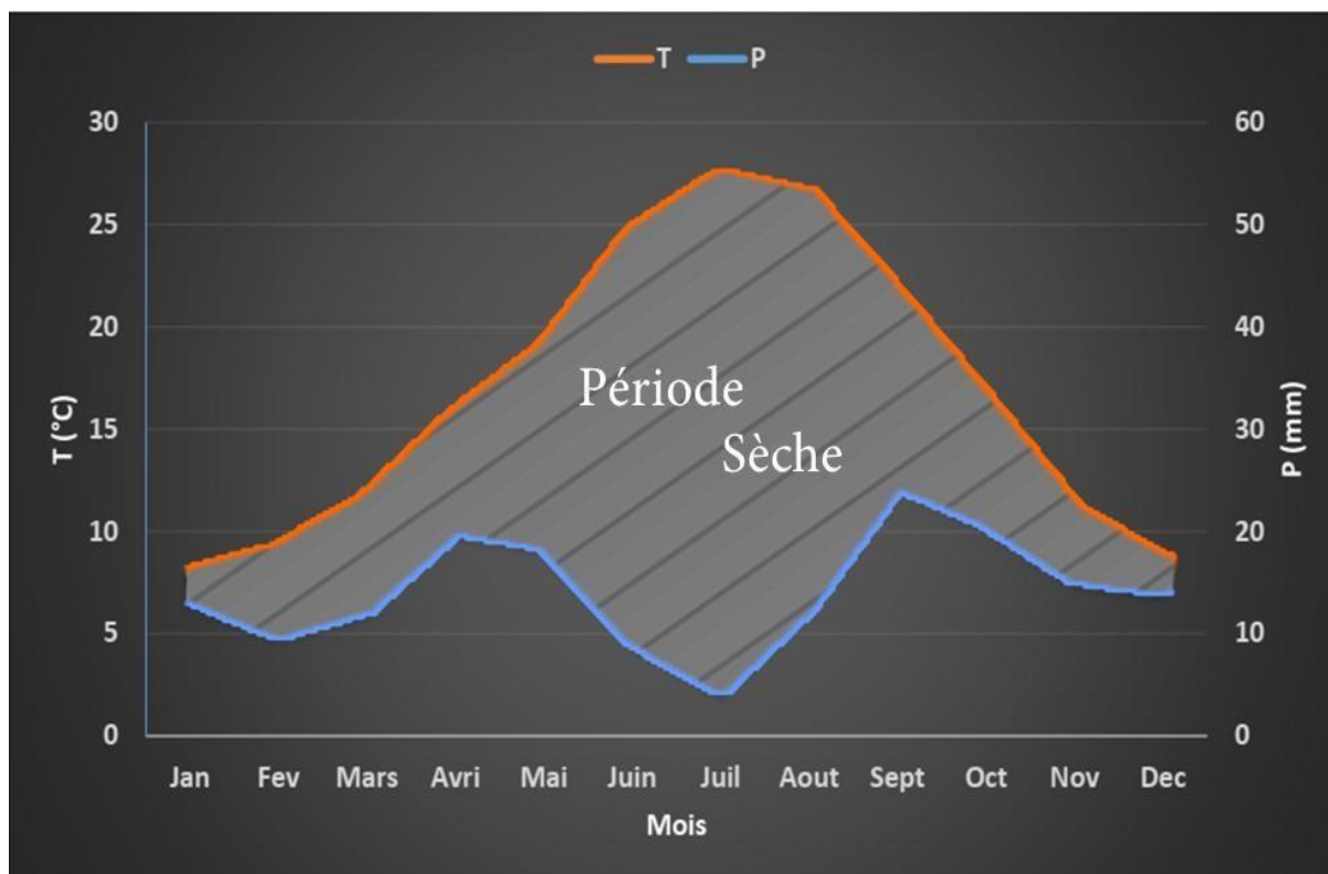
Figure n°11: Diagramme ombrothermique de la région étudiée (1994-2016).
