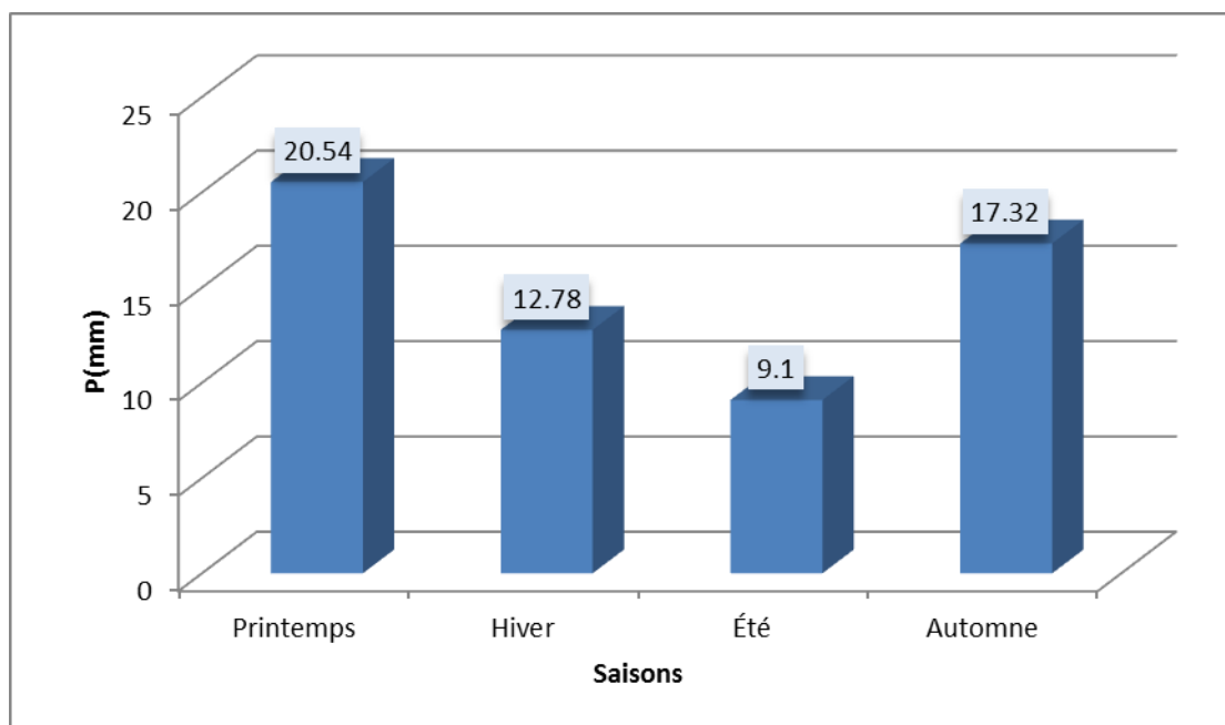
Figure n°06 : Régime saisonnier des précipitations (en mm) de la région d'étude (1994-2016).
