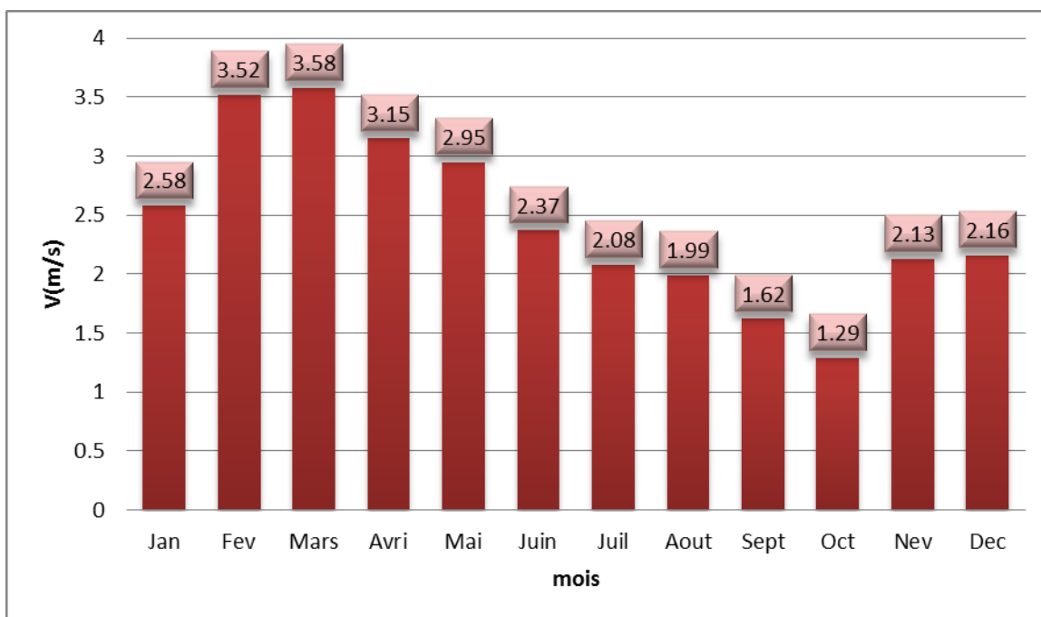
Figure n°07: Vitesse annuelle moyenne des vents de la région d'étude (2004-2016).
