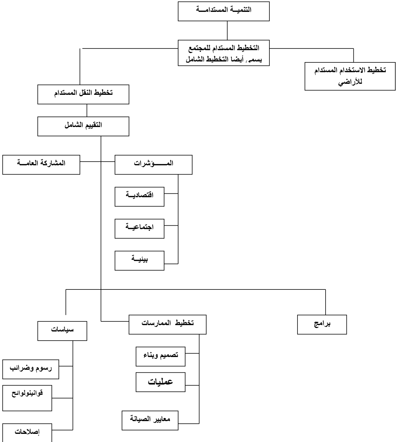
الشكل رقم (03): استدامة عملية التخطيط
