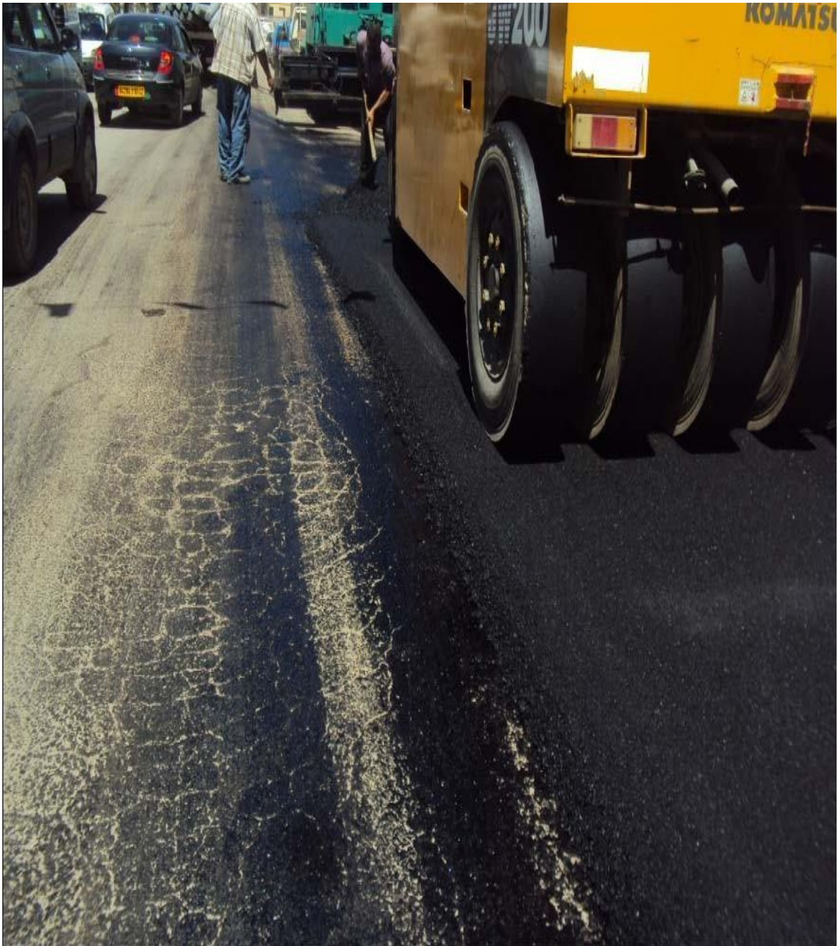
Figure AI.7 photographie de mise en œuvre de béton bitumineux dans la chaussée
