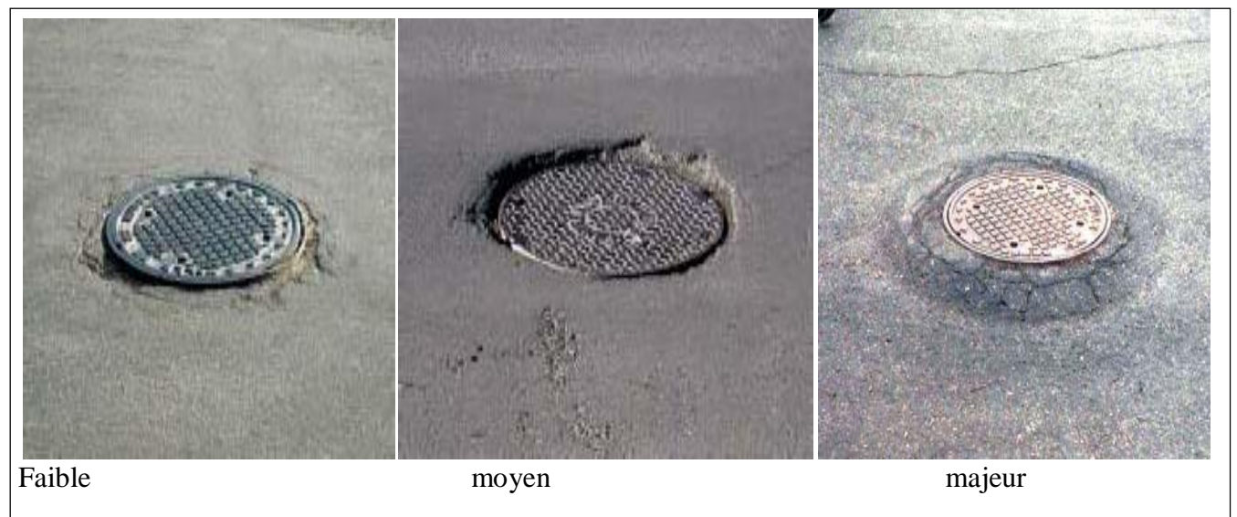
b. Dénivellation des regards
