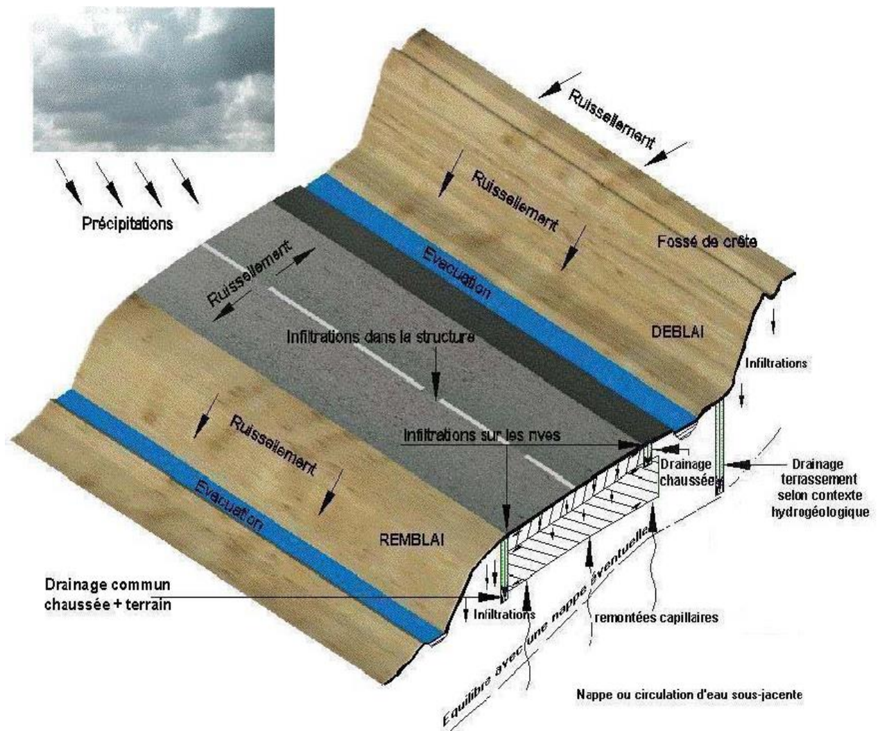
Figure III.1 récupération et évacuation de l'eau dans une chaussée (SETRA : guide technique de drainage routier, janvier 2009)
