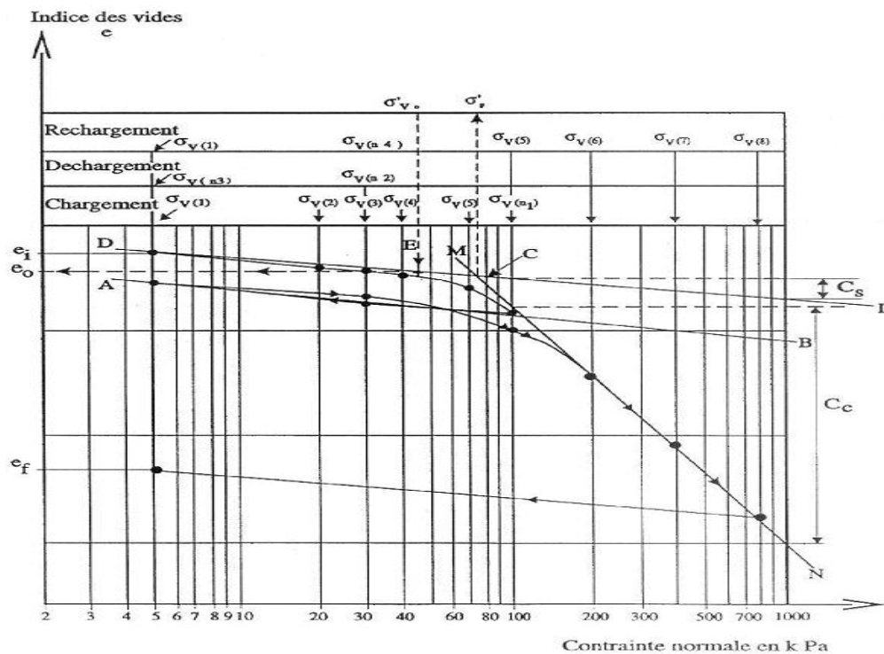
Figure II.13 Principe d'interprétation des courbes de compressibilité par les méthodes d'essais LPC (Magnan et al., 1985).
