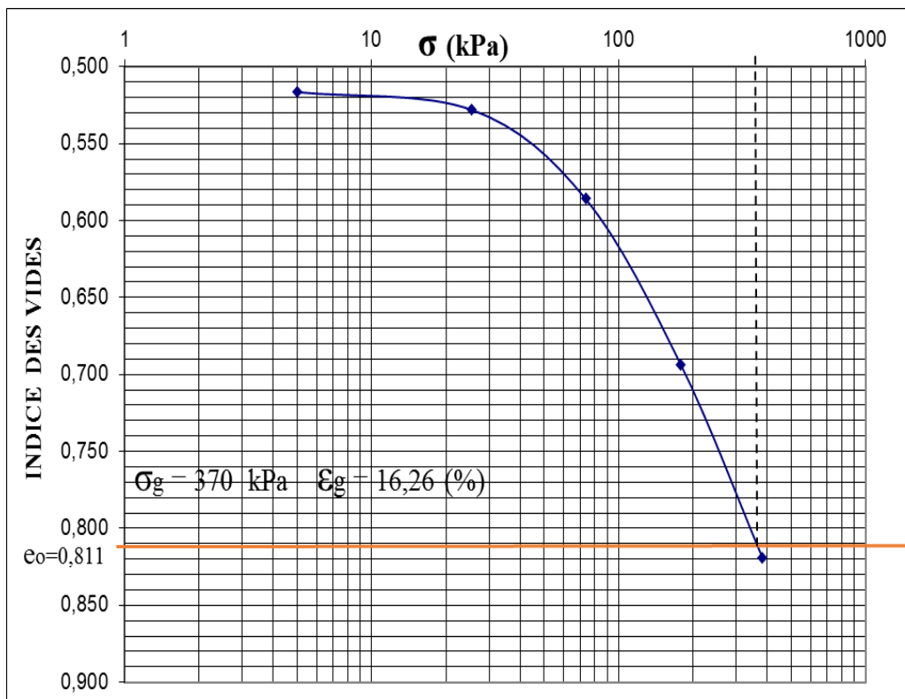
Figure III-30 : Essai de gonflement n° 3 (méthode du CEBTP.).
