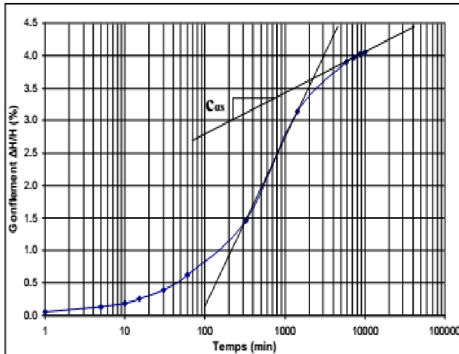
Figure II.17 : Courbes de gonflement.
