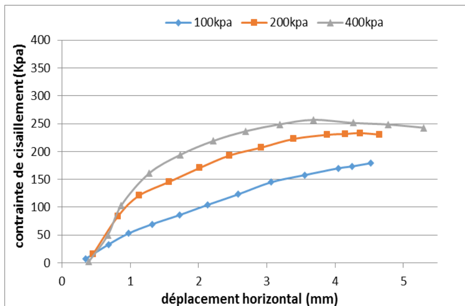
Figure III-16- courbe contrainte/déformation N°2.
