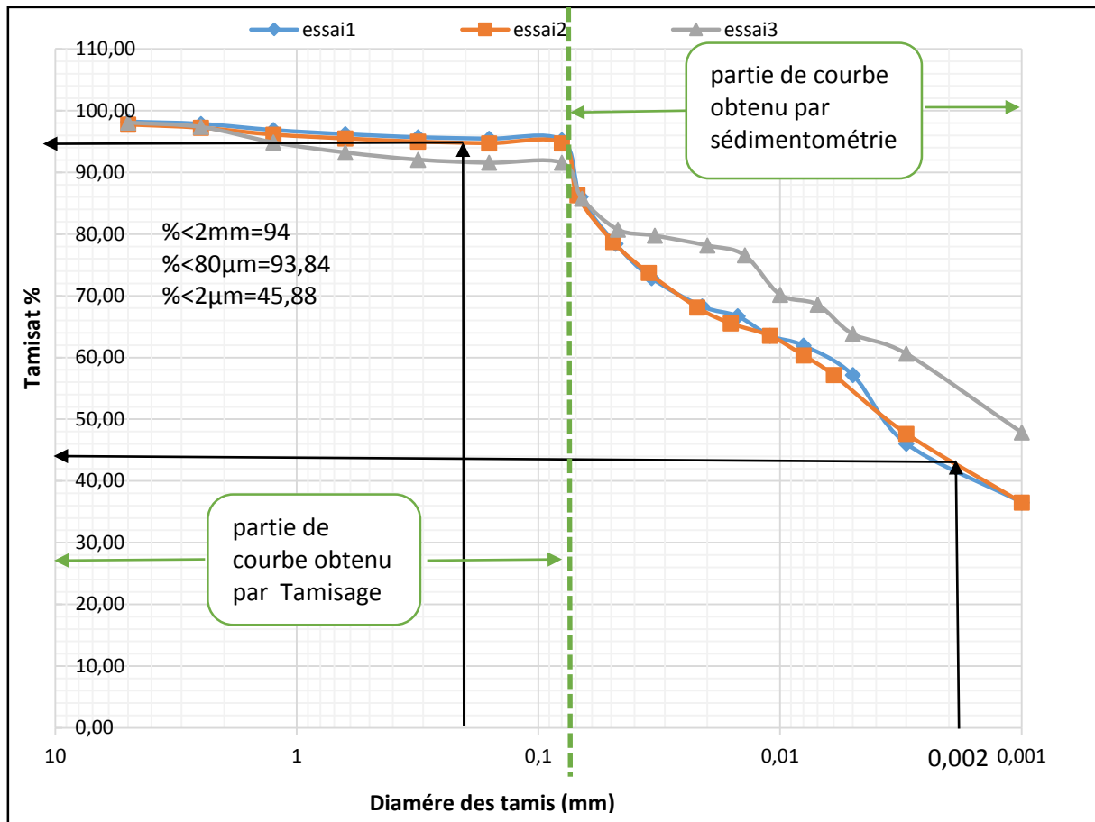
Figure III-1- Courbe d'analyse granulométrique (tamisage et sédimentométrie).
