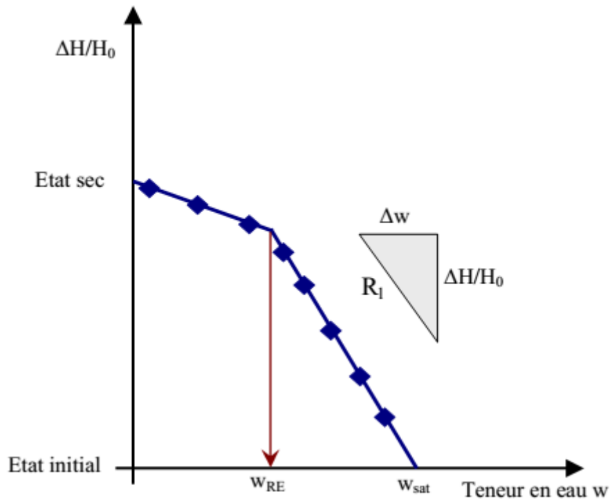
Figure II.18: Principe d'interprétation des courbes de dessiccation à partir des essais de dessiccation conformes à la norme AFNOR.
