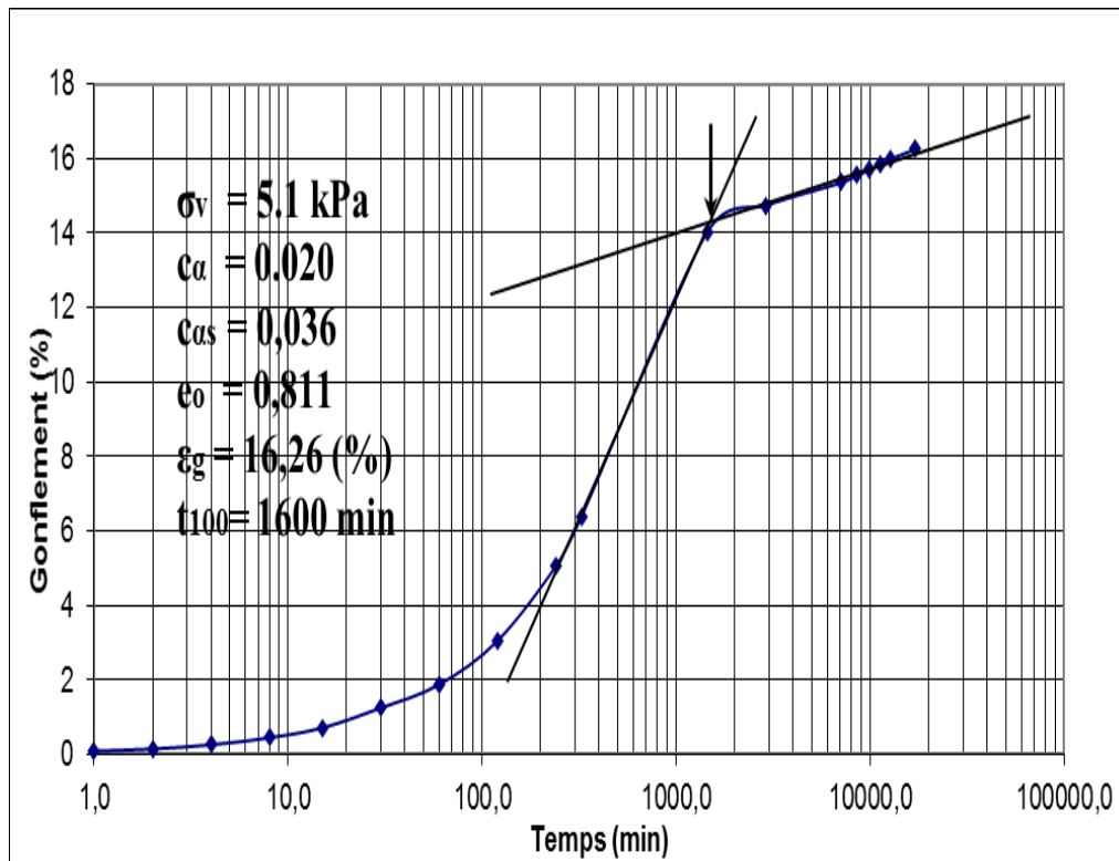
Figure III-33 : Essai de gonflement n° 3 \Delta H/H_0 on fonction de \log t (méthode du CEBTP).
