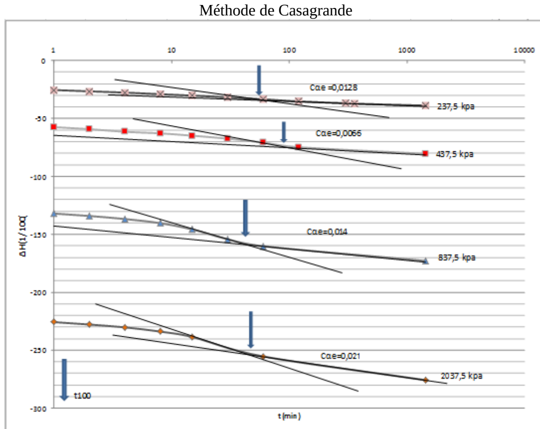
Figure III-27 Courbe de consolidation (essai n° 2).
