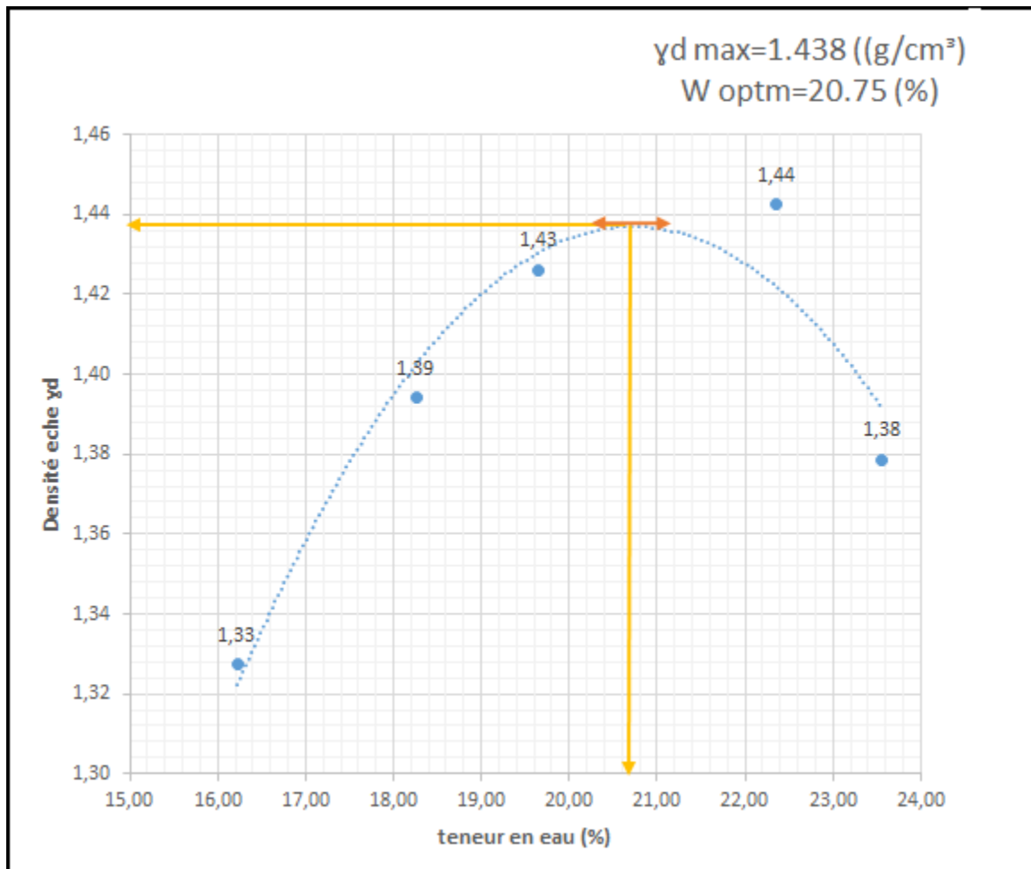
Figure III-5- Courbes d'essais Proctor normal.
