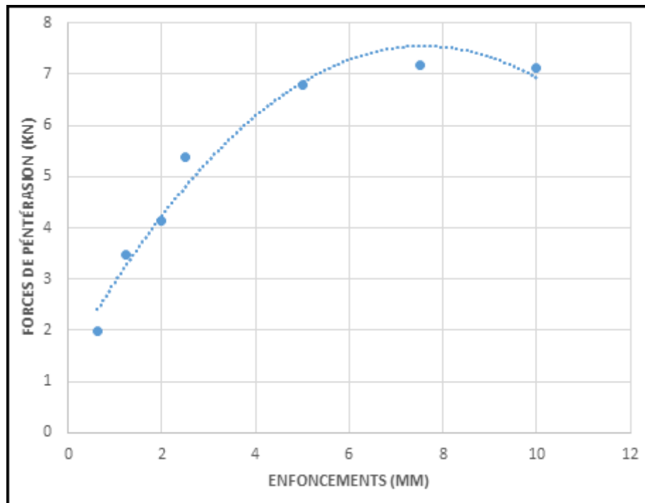
Figure III- 8- Courbe d'essai de C.B.R immédiat N°3.
