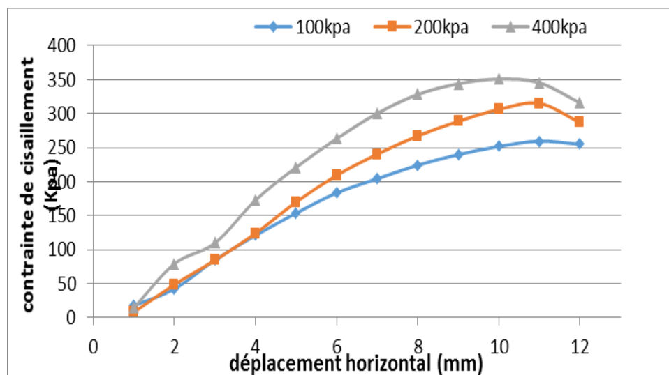
Figure III-17- courbe contrainte/déformation N°3.
