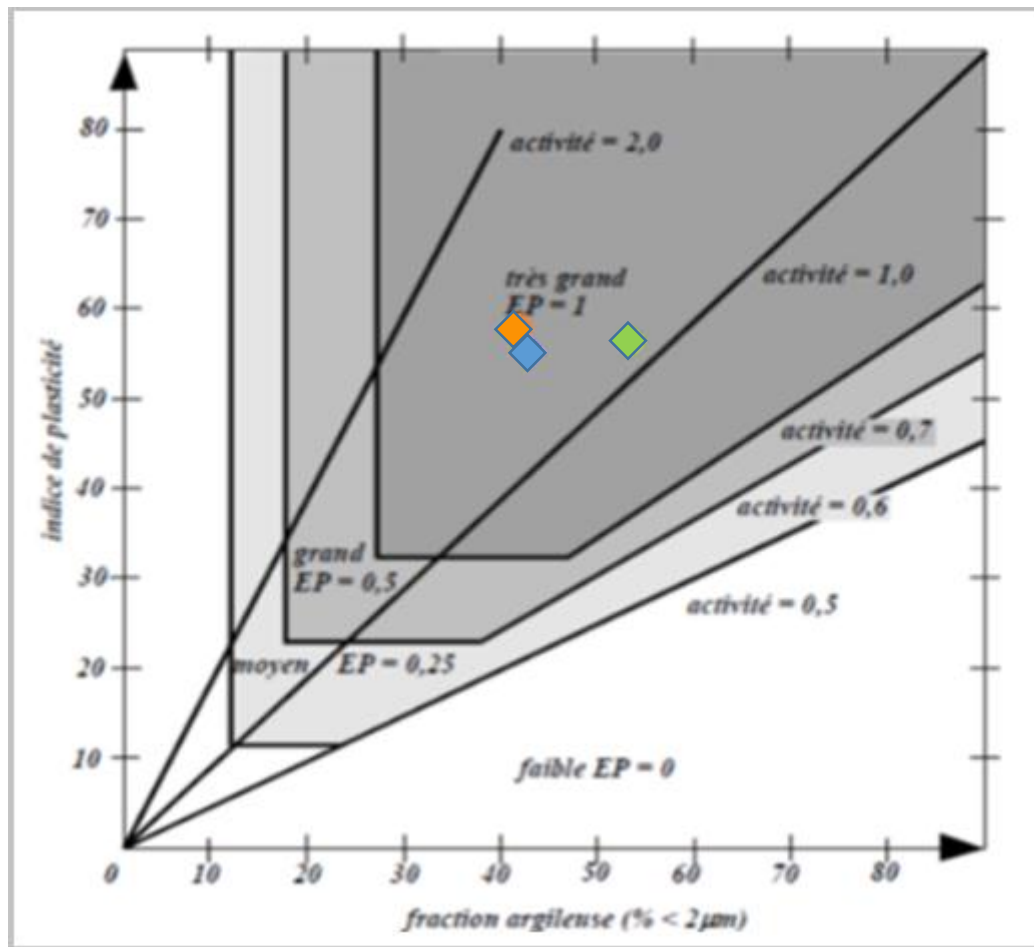
Figure III-39: Classification du sol étudié (Williams et Donaldson (1980)).
