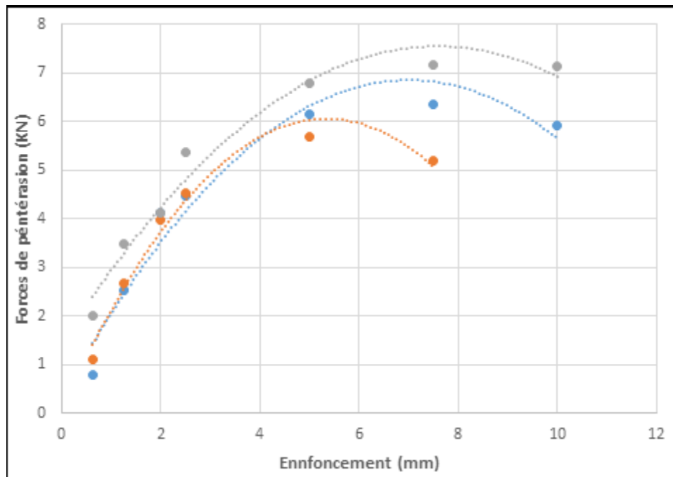
Figure III- 9- Courbes des essais des C.B.R immédiat.
