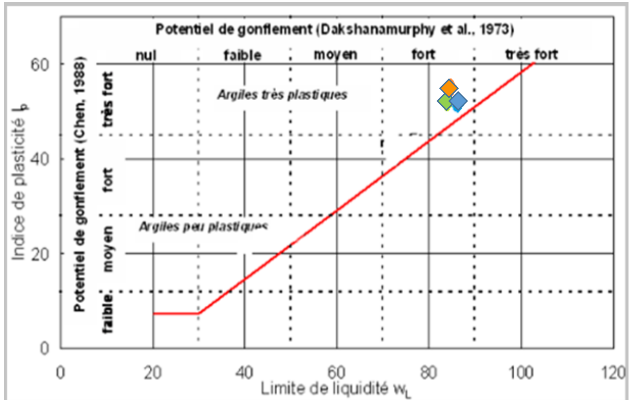
Figure III-36: Courbes de limites d'Atterberg de la série d'essai N°(1+2+3)
