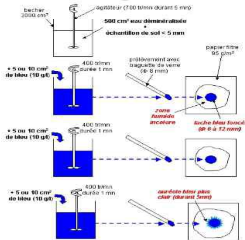
Figure II.5 : Les étapes de l'essai au bleu de méthylène.
