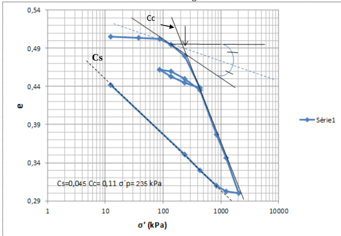
Figure III-19 Courbe de compressibilité (essai n° 1).
