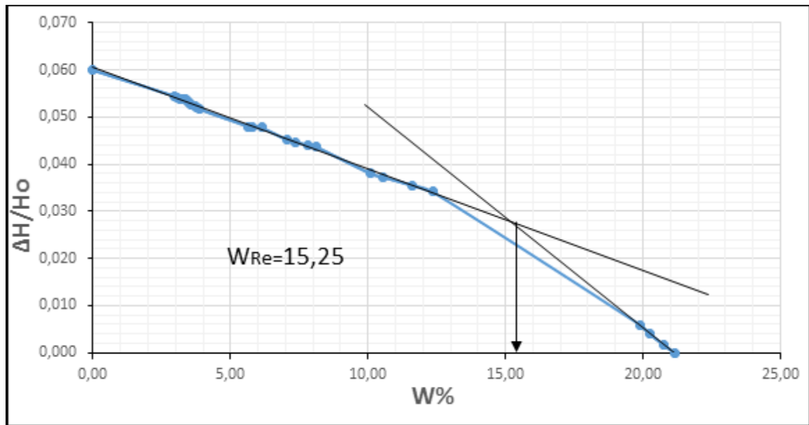
Figure III-34 Essai de dessiccation sur échantillon non remanié n° 1.
