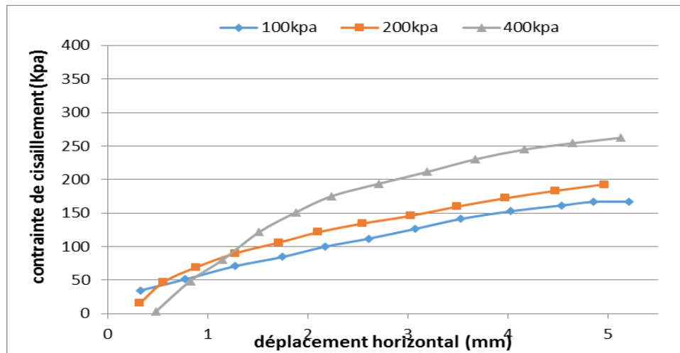
Figure III-15- courbe contrainte/déformation N°1.
