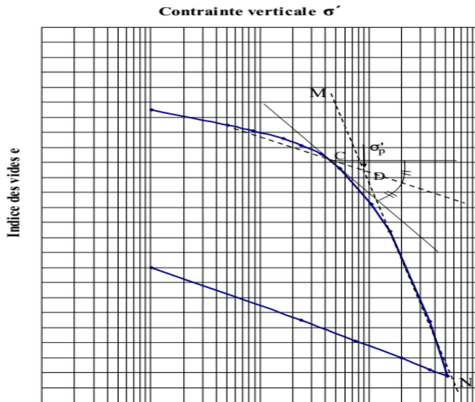
Figure II.15 Principe d'interprétation des courbes de compressibilité par la méthode classique de Casagrande.
