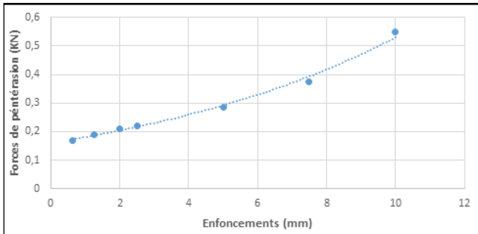
Figure III- 11- Courbe d'essai de C.B. imbibition N°2.
