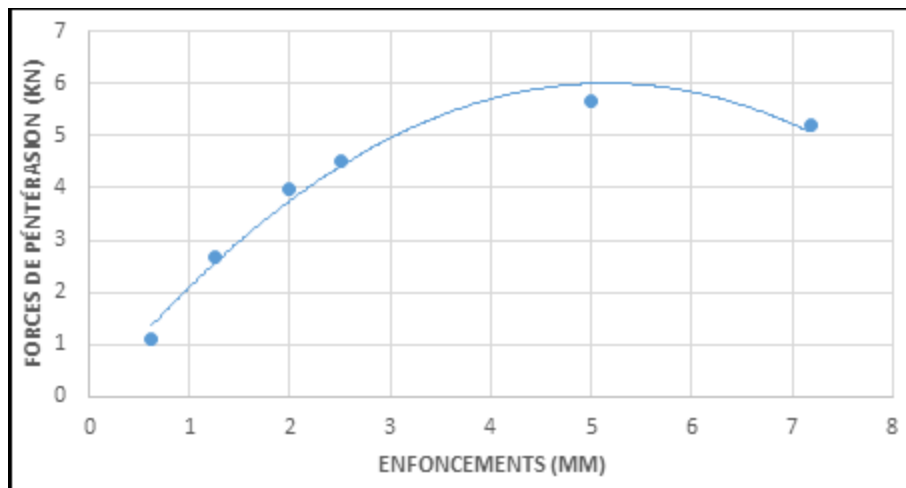
Figure III- 7- Courbe d'essai de C.B.R immédiat N°2.
