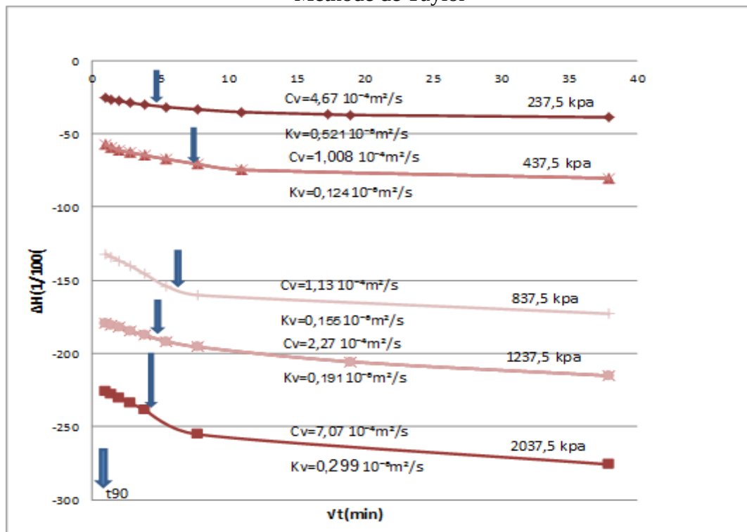
Figure III-26 Courbe de consolidation (essai n° 2).
