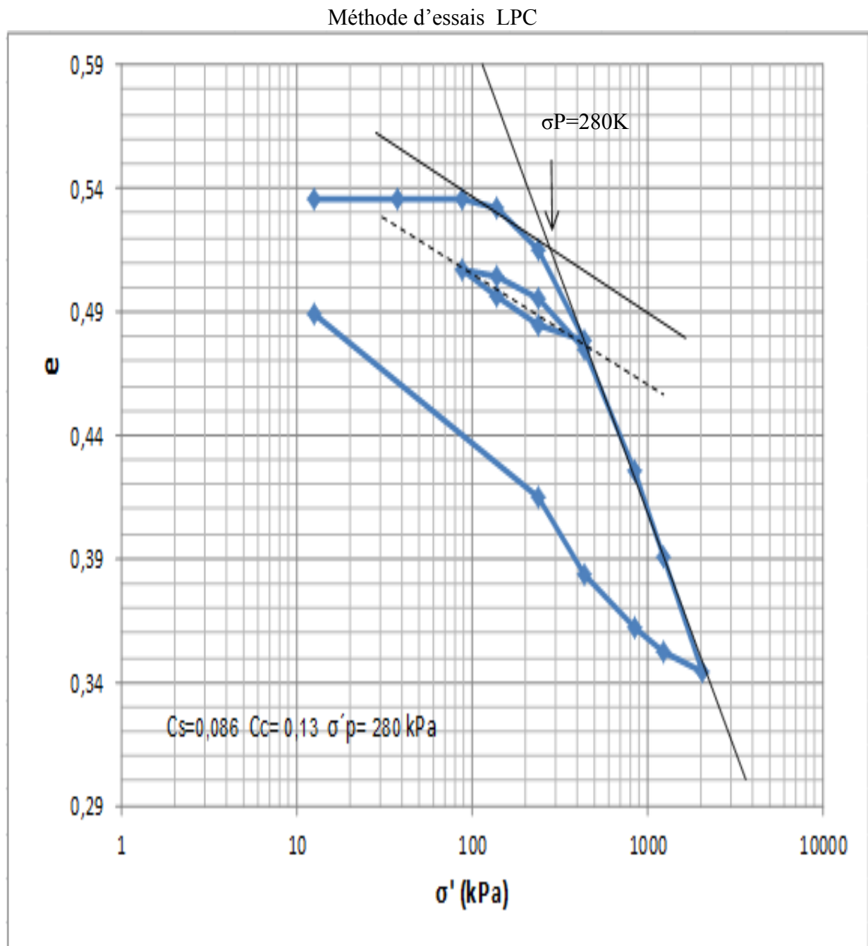
Figure III-23 Courbe de compressibilité (essai n° 2).
