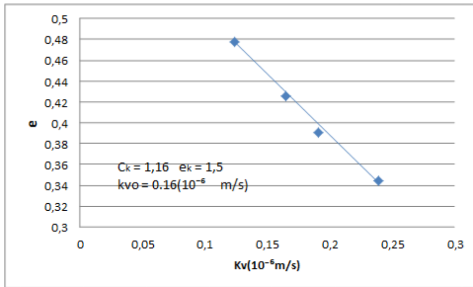
Figure III-25 Courbe de perméabilité (essai n° 2).
