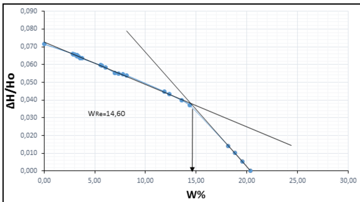
Figure III-35 Essai de dessiccation sur échantillon non remanié n° 2.
