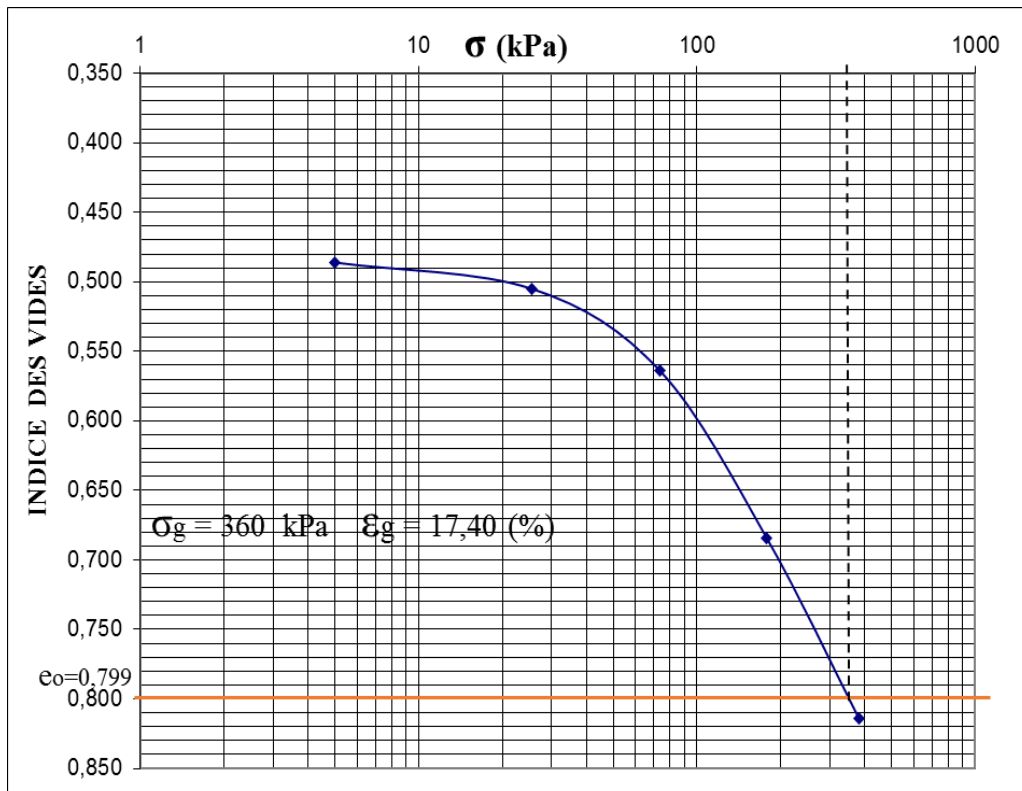
Figure III-29 : Essai de gonflement n° 2 (méthode du CEBTP).
