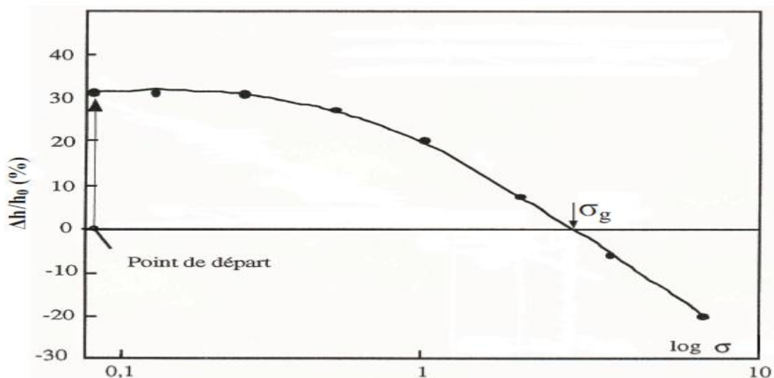
Figure I-14 : Essais de gonflement libre [4].
