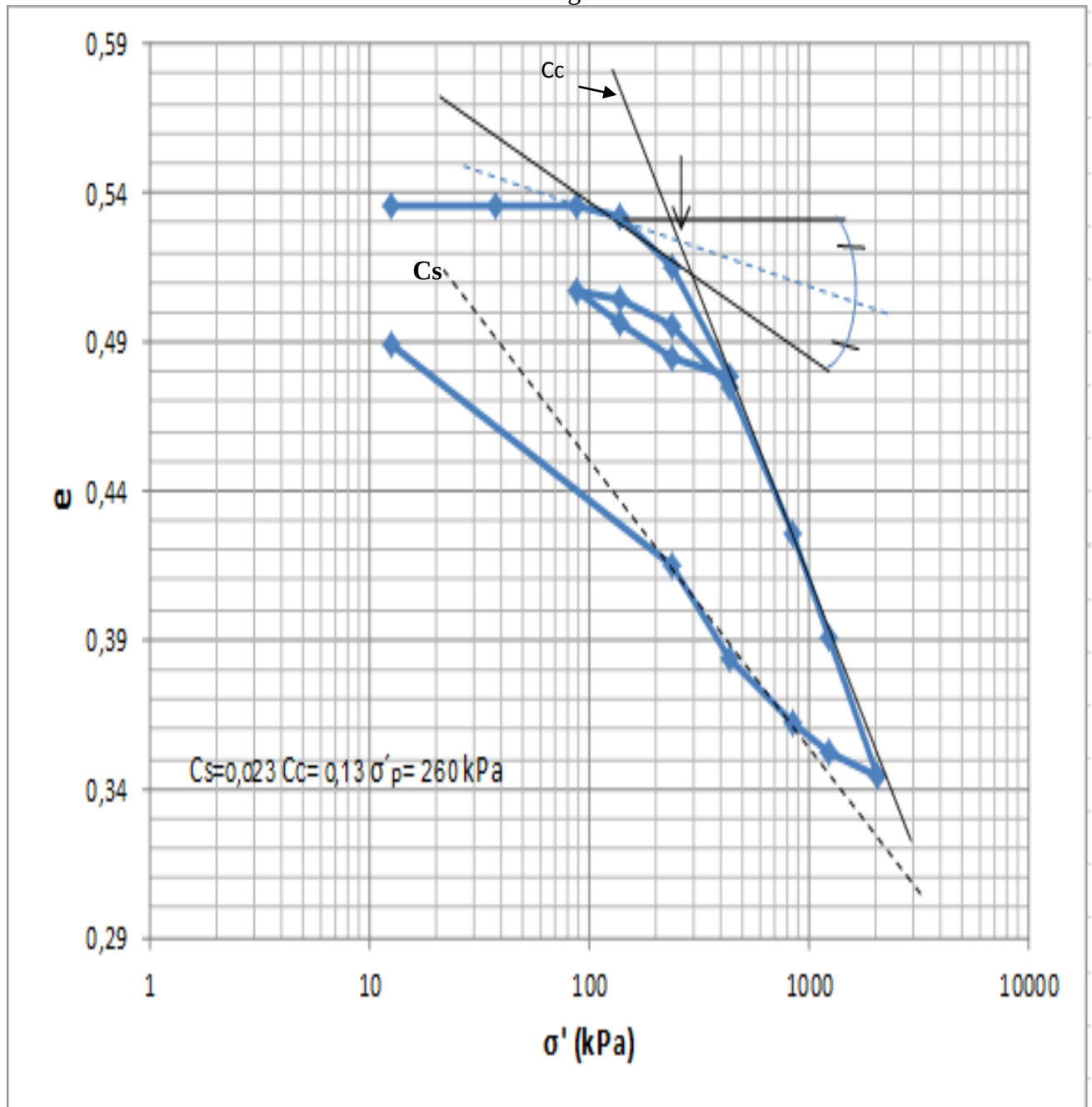
Figure III-24 Courbe de compressibilité (essai n° 2).
