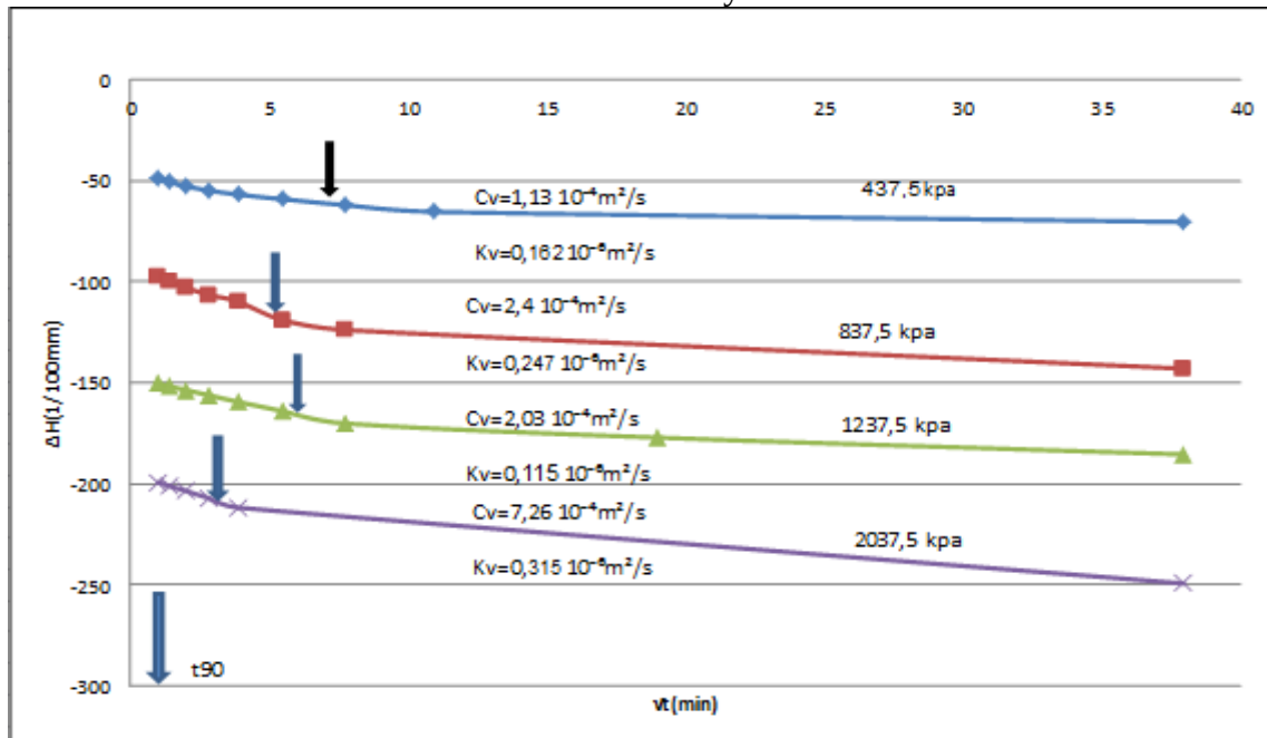
Figure III-21 Courbe de consolidation (essai n° 1).
