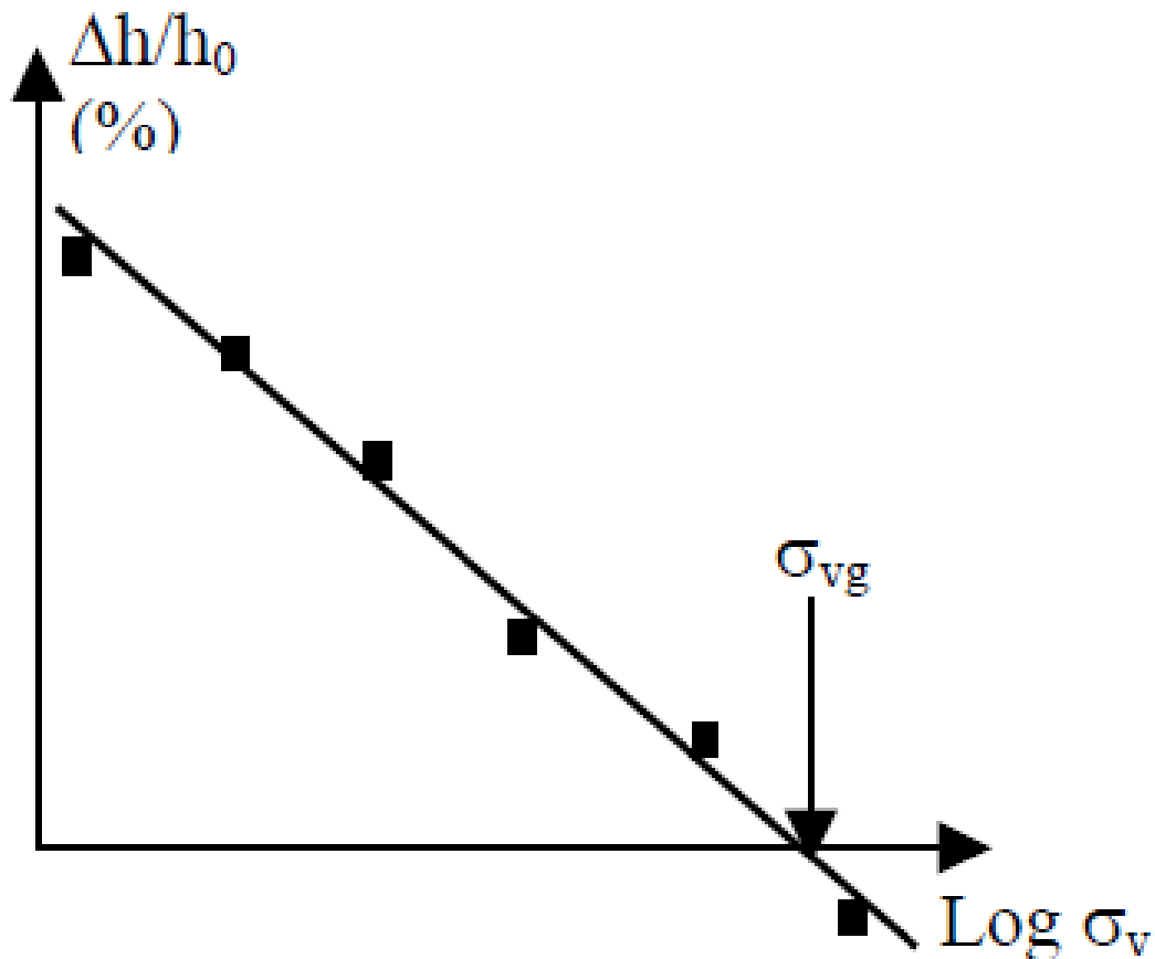
Figure I-15 : Essais de gonflement en parallèle [4].
