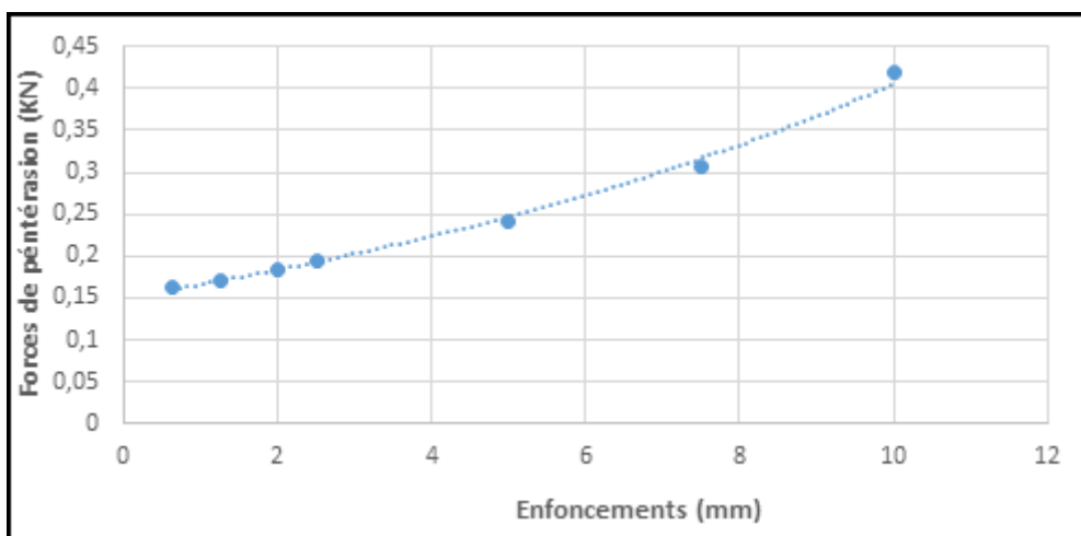
Figure III- 12- Courbe d'essai de C.B. imbibition N°3.
