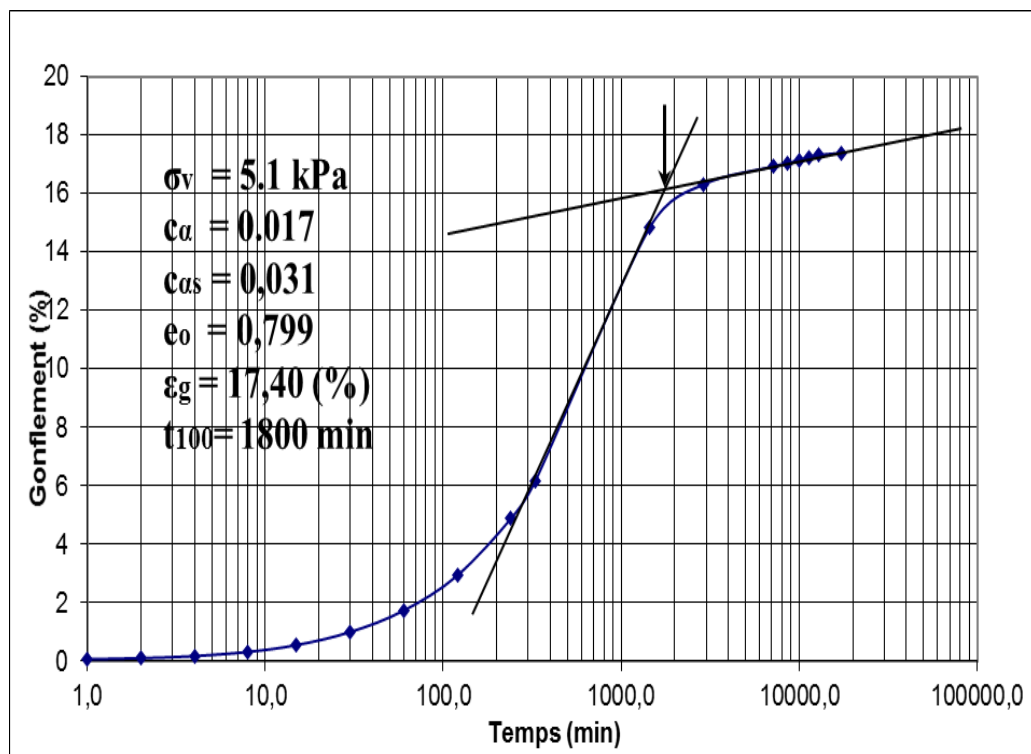
Figure III-32 : Essai de gonflement n° 2 \Delta H/H_o on fonction de \log t (méthode du CEBTP).
