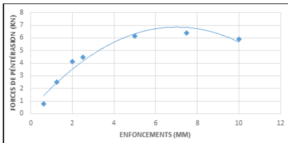
Figure III- 6- Courbe d'essai de C.B.R immédiat N°1.
