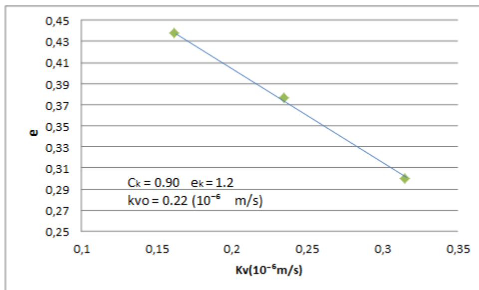
Figure III-20 Courbe de perméabilité (essai n° 1).
