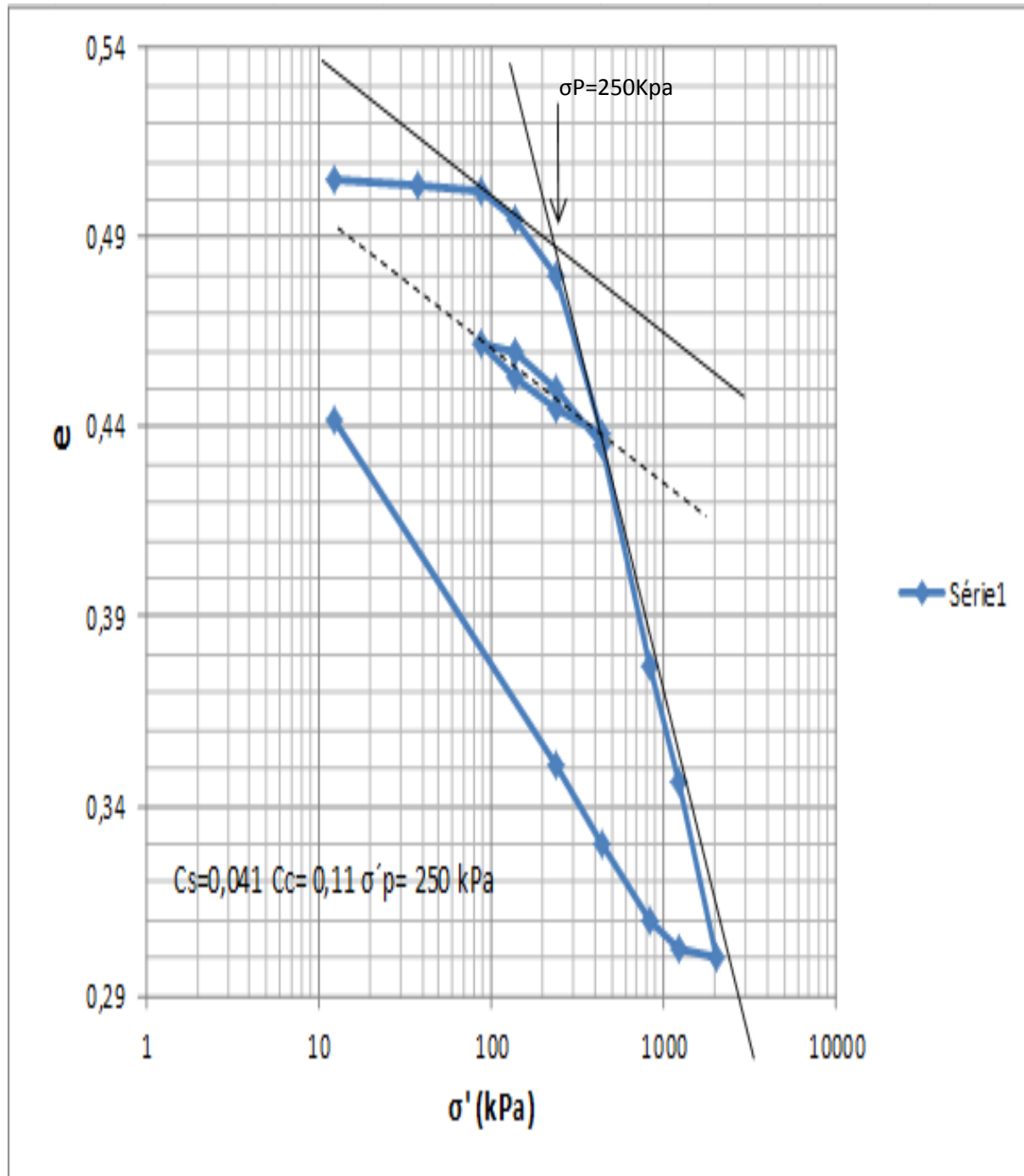
Figure III-18 Courbe de compressibilité (essai n° 1).
