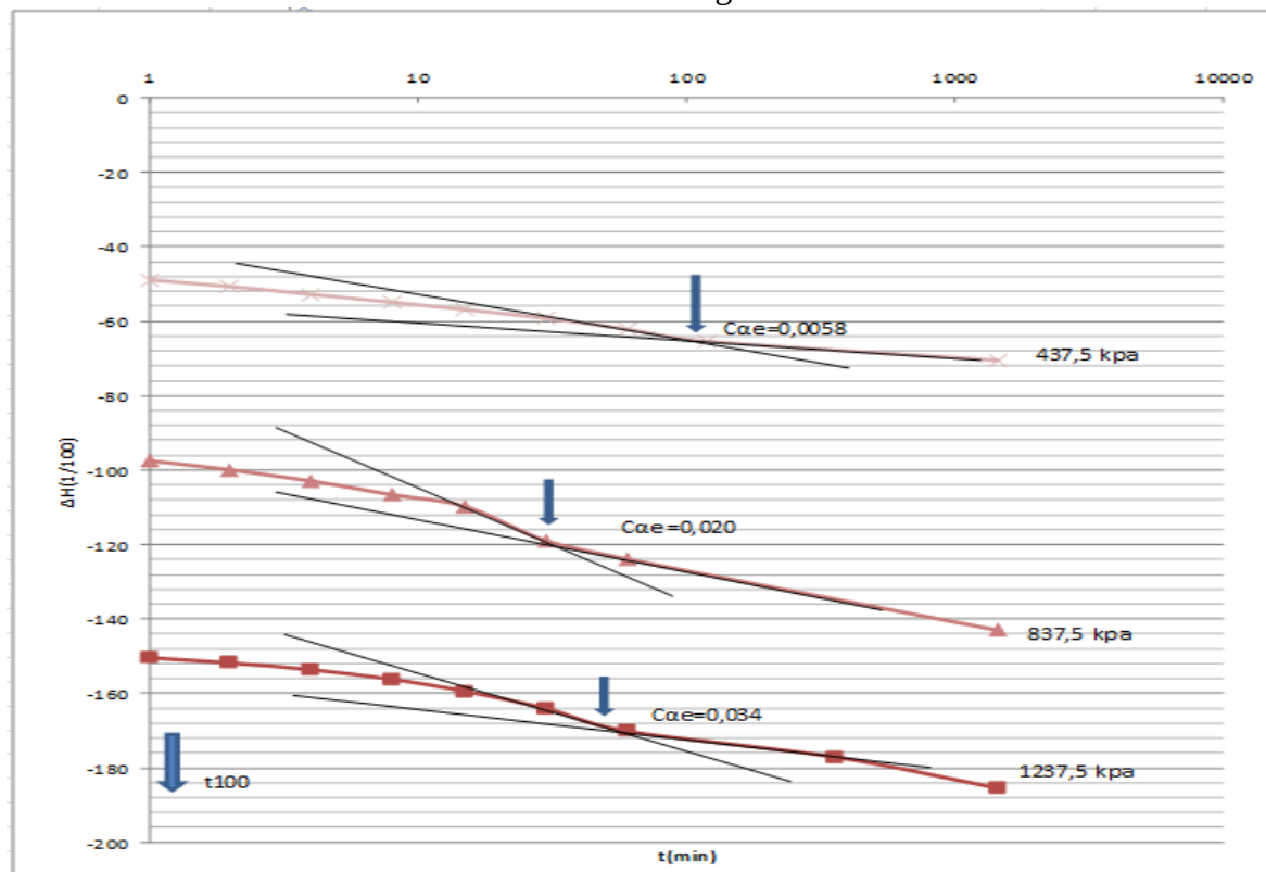
Figure III-22 Courbe de consolidation (essai n° 1).
