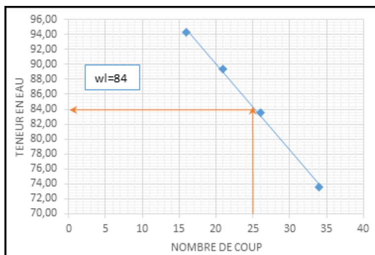
Figure III-2- Les courbes et la valeur de limite liquidité l'essai N°1.
