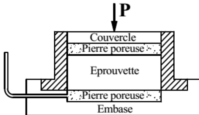
Figure II.12: Coupe schématique d'une cellule œdométrique conventionnelle à chargement par poids.
