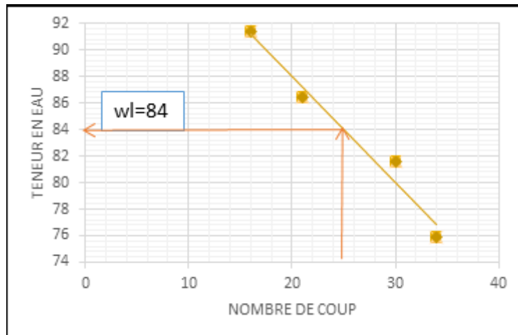
Figure III-3- Les courbes et la valeur de limite liquidité l'essai N°2.
