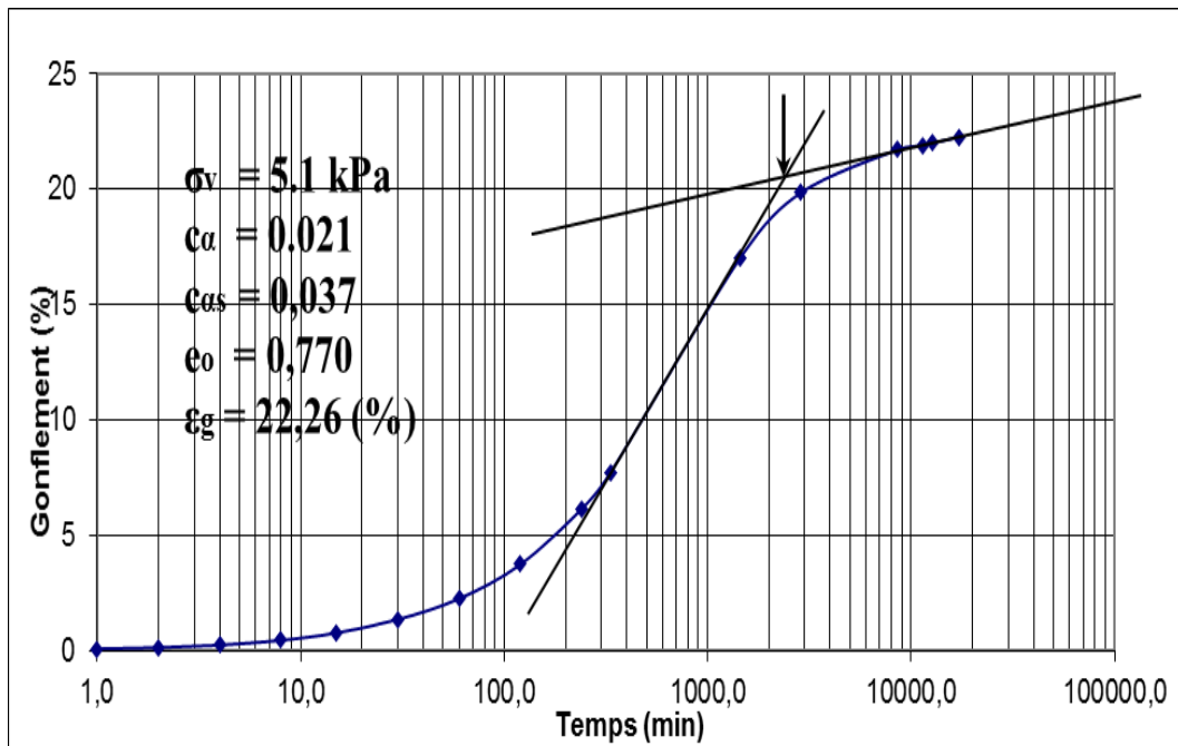
Figure III-31 Essai de gonflement n°1 \Delta H/H_o on fonction de \log t (méthode du CEBTP)
