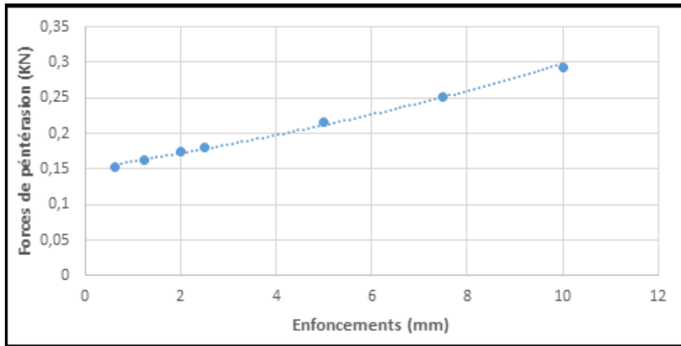
Figure III- 10- Courbe d'essai de C.B. imbibition N°1.
