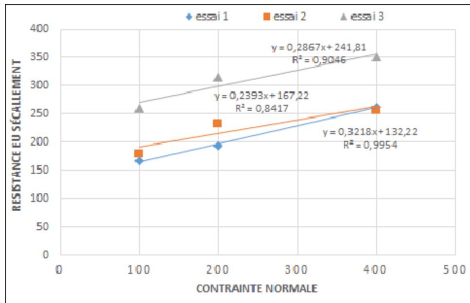
Figure III-14- Courbe d'essai cisaillement direct.
