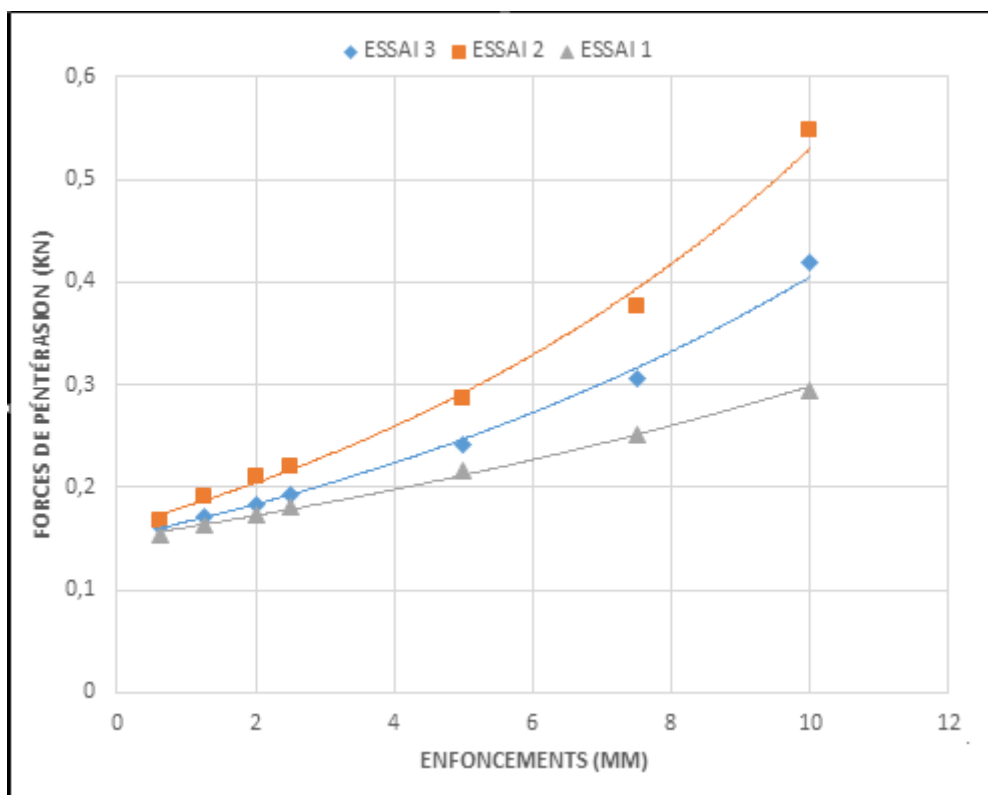
Figure III -13- Courbes des essais des C.B.R imbibition.
