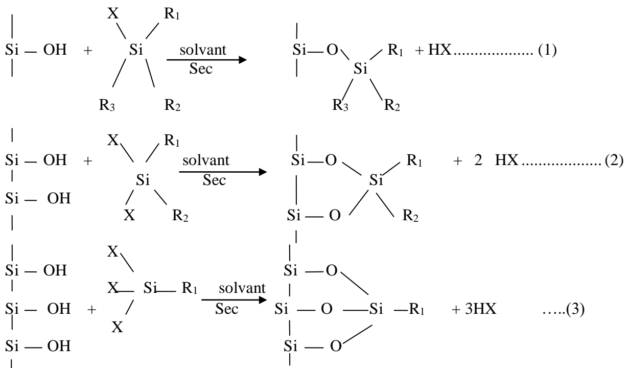
Figure I.7 : Schéma possibilités de modification d'une surface argileuse par un monomère (1) : monofonctionnel, (2) : di fonctionnel et (3) : trifonctionnel [60].
