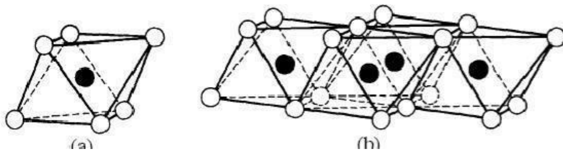
Figure I.2 : Schéma (a) d'un octaèdre d'aluminium et (b) d'une couche octaédrique d'après Grim (1968) [28].
