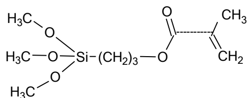
Figure.II.2 : Schéma de formule chimique de TriMéthoxysilylpropylméthacrylate.
