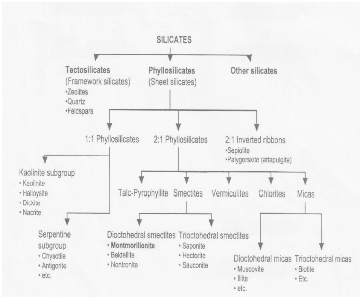
Figure I.3 : Classification des principales catégories d’argiles (Manas-Zloczower 1994).
