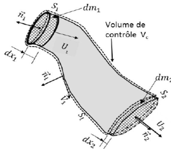
Figure III.3: Tube de lignes de courant d'un fluide
