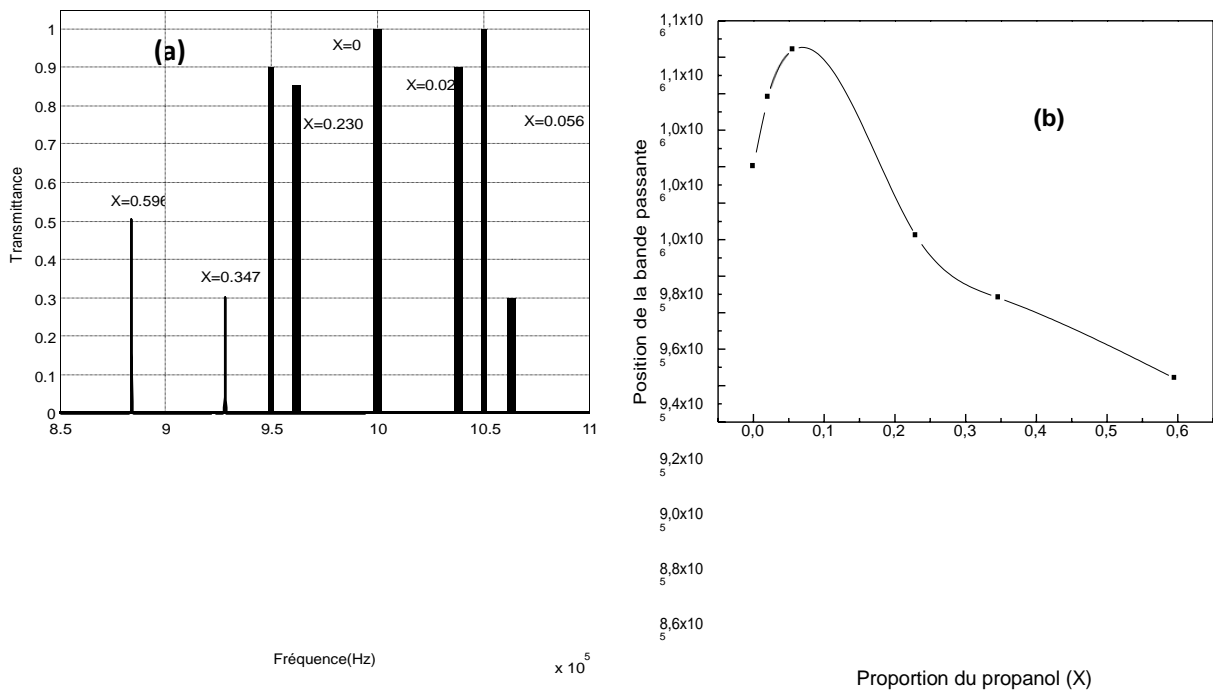
Figure III.17: (a) Spectre de transmission en fonction de la fréquence pour différentes concentrations du propanol, (b) : évolution de la fréquence de résonance en fonction le pourcentage du propanol
