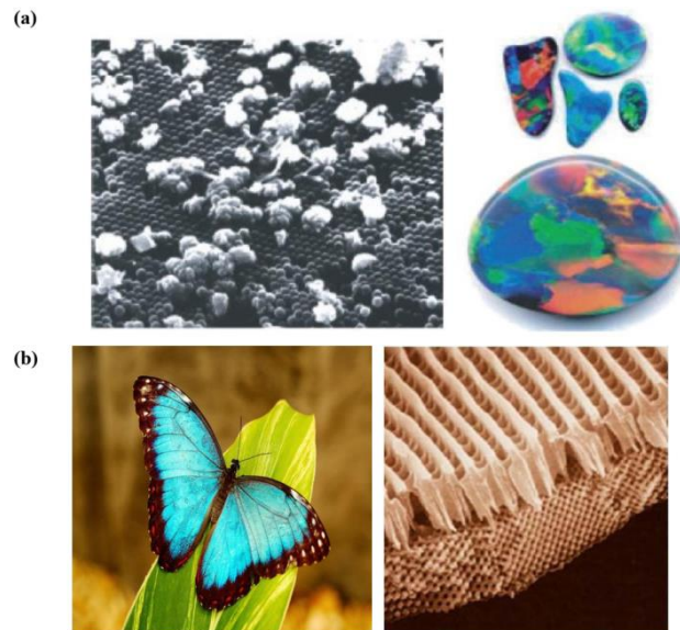
Figure II.3 Exemples de cristaux photoniques naturels : (a) Photographies d'opales à différentes échelles [51], (b) Photographies des ailes de papillon [52].
