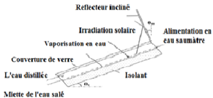
Figure II. 5 - Réflecteur externe supérieur avec un distillateur solaire à mèche incliné [12].
