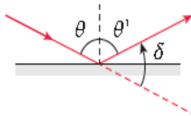
Figure I.3. L'angle de déviation d'un rayon lumineux.
