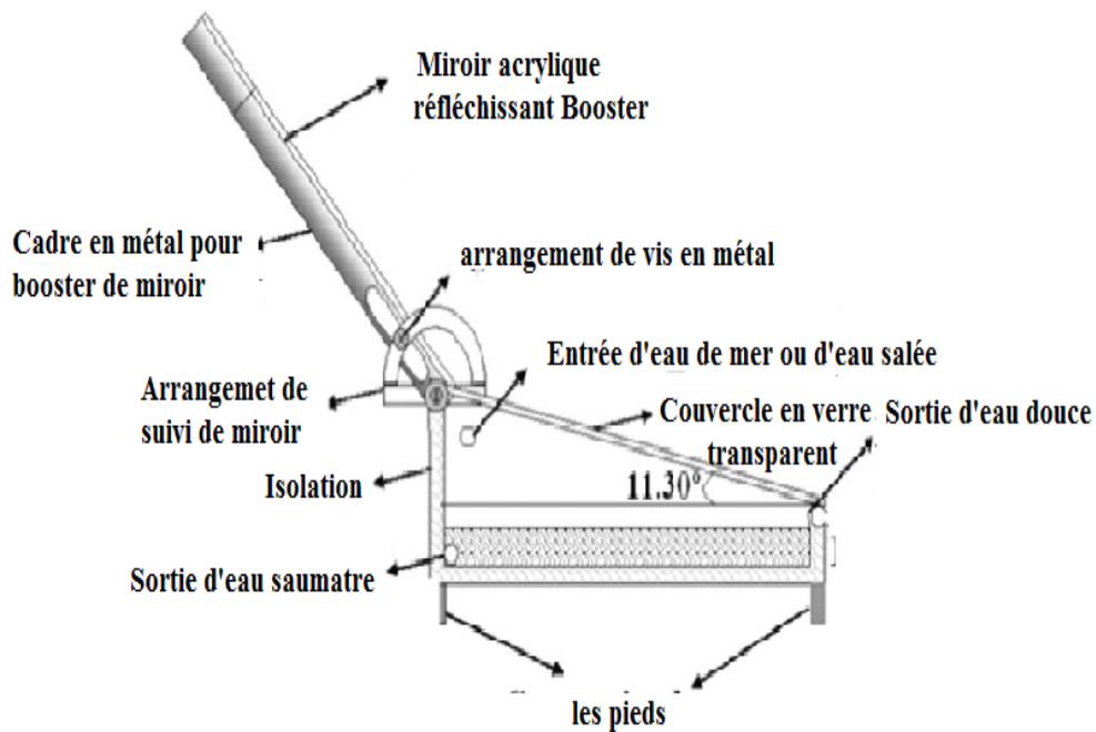
Figure II.10 - Vue de l'unité de distillation solaire avec un miroir [12].
