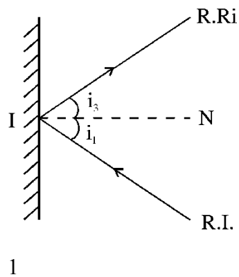
Figure I.2- représente schématiquement un miroir plan.
