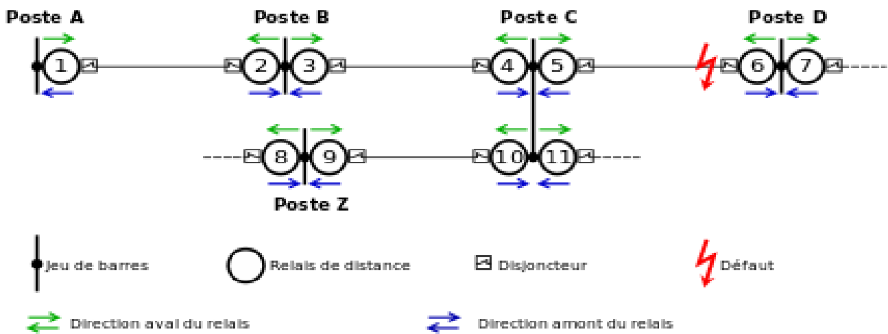
Figure.II.1. les zones de protection d'un réseau électrique. [9]
