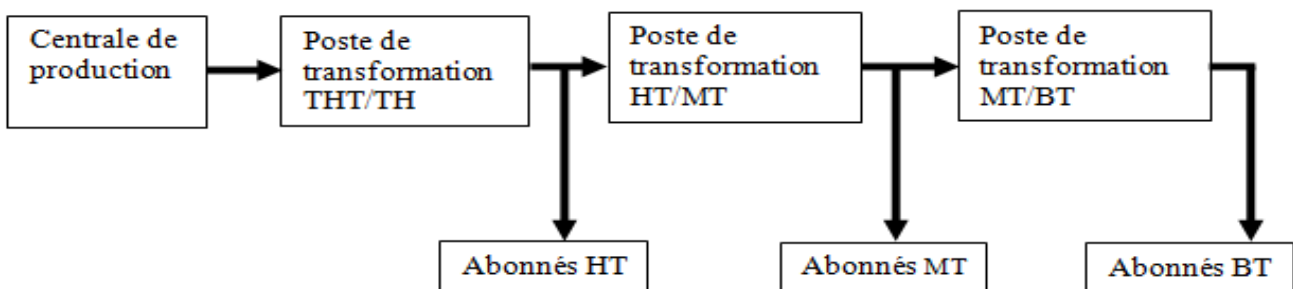
Figure. I.1. schémas générale du réseau électrique. [2]
