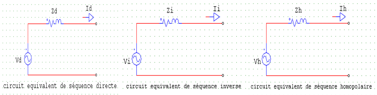
Figure.III.2. Circuit équivalent des séquences.
