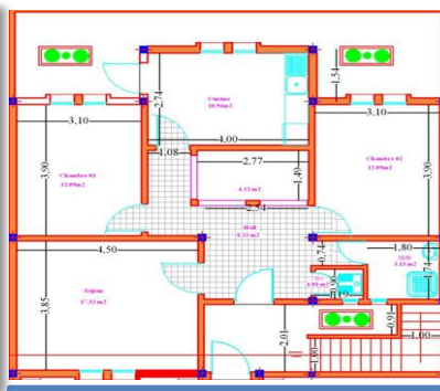
الشكل رقم (18) : مخطط تفصيلي
